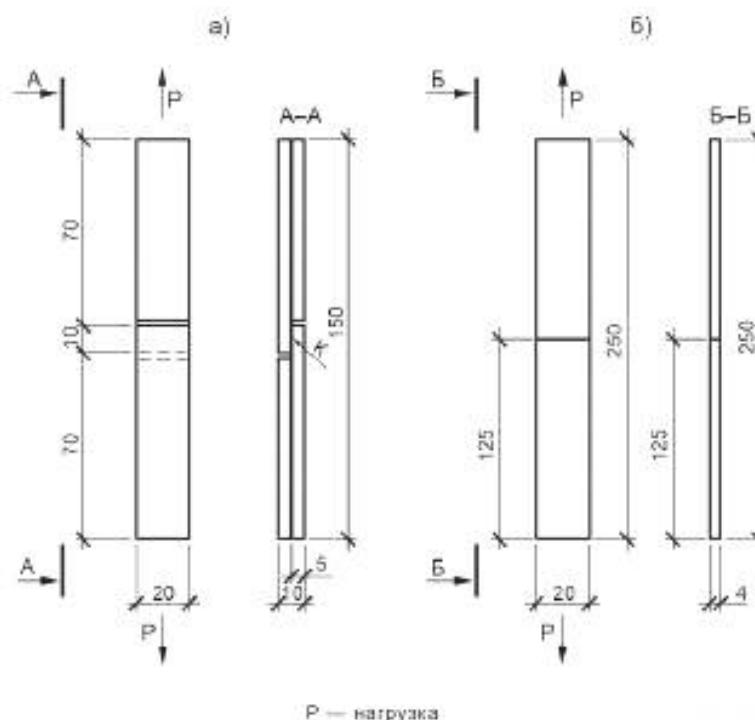
Рисунок 1 — Схемы приложения нагрузки при испытаниях на скалывание при растяжении (а) и на растяжение клеевого торцевого соединения впрыток (б) соединения впрыток.
