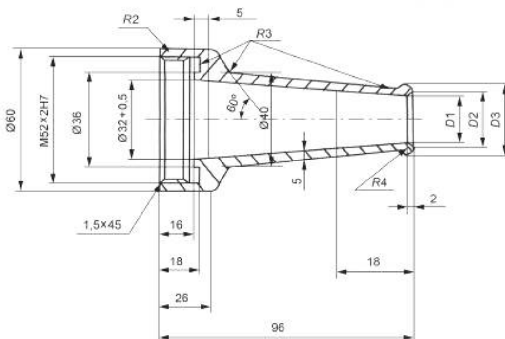
Рисунок Б.2 — Мерные насадки для ствола-водомера
