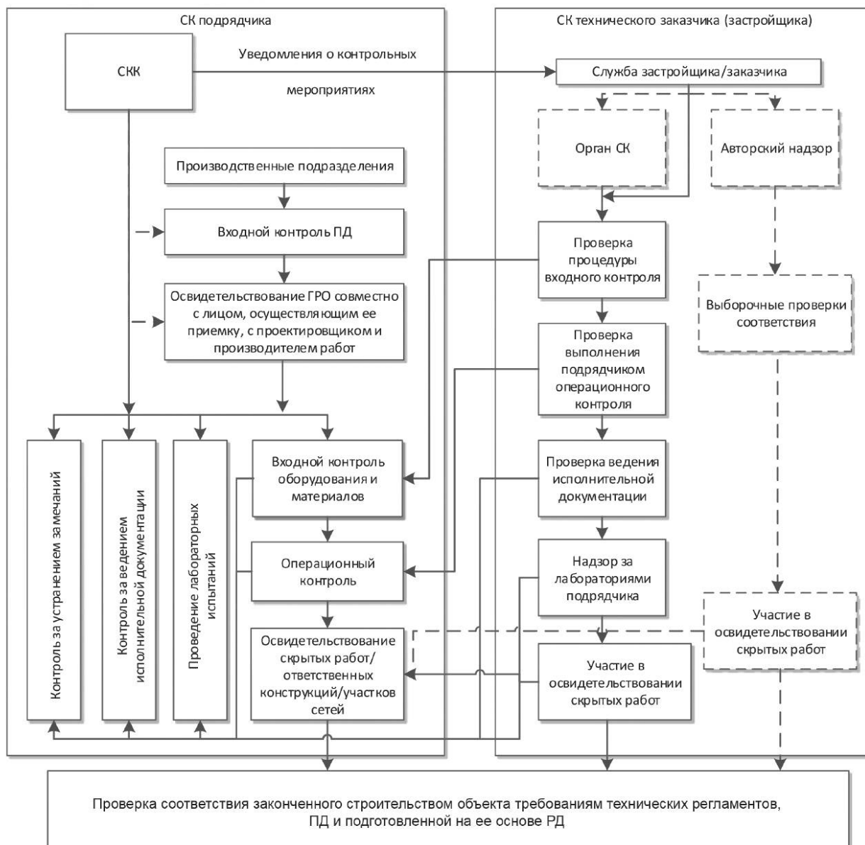
Рисунок 1 — Схема осуществления СК
