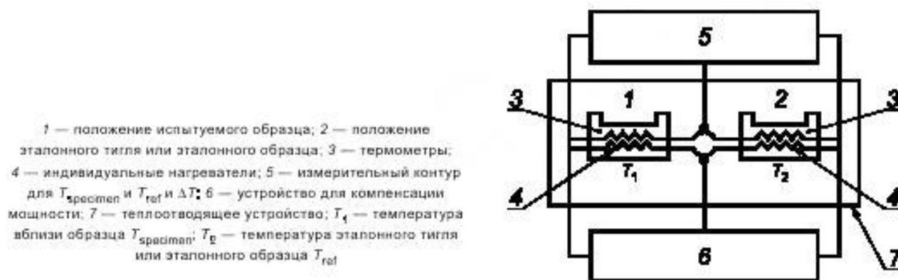
Рисунок ДА.3 — Схема прибора ДСК с компенсацией мощности
