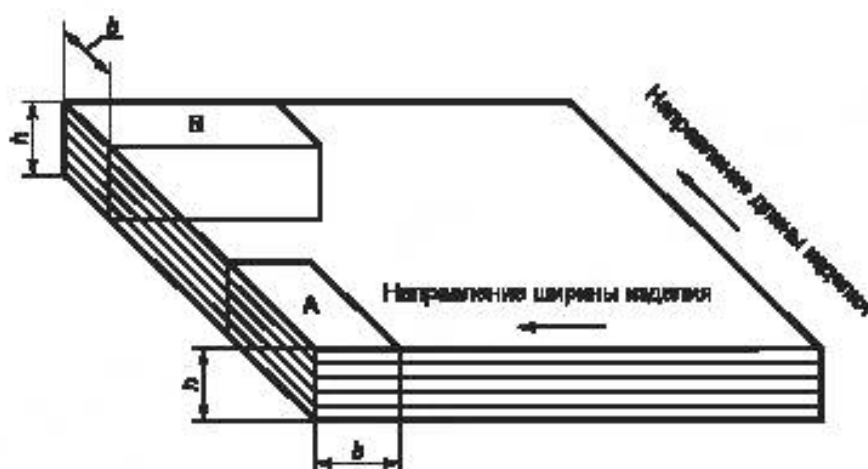
Рисунок ДА.4 — Схема формирования (вырезания) образцов
