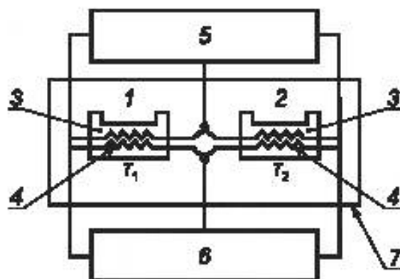
1 — положение испытуемого образца; 2 — положение эталонного тигля или эталонного образца; 3 — термометры; 4 — индивидуальные нагреватели; 5 — измерительный контур для T_{specimen} и T_{ref} и \Delta T ; 6 — устройство для компенсации мощности; 7 — теплоотводящее устройство; T_1 — температура вблизи образца ( T_{specimen} ); T_2 — температура эталонного тигля или эталонного образца ( T_{ref} )
