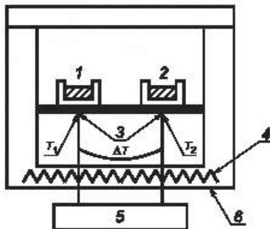
1 — испытуемый образец; 2 — эталонный тигель или эталонный образец; 3 — термолары; 4 — общий нагреватель; 5 — измерительный контур для T_{specimen} , T_{ref} и \Delta T ; 6 — печь; T_1 — температура испытуемого образца ( T_{specimen} ); T_2 — температура эталонного тигля или эталонного образца ( T_{ref} ); \Delta T — разность температур испытуемого образца и эталонного тигля или эталонного образца
