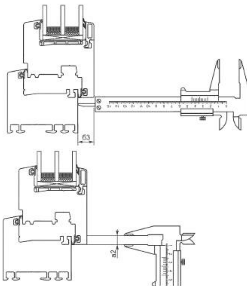
Рисунок Г.6 — Определение величины рабочего наплыва створки
