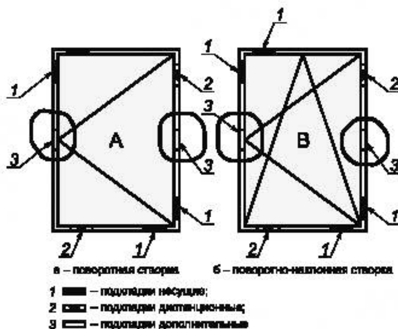
Рисунок Г.10 — Схема расположения установочных подкладок
