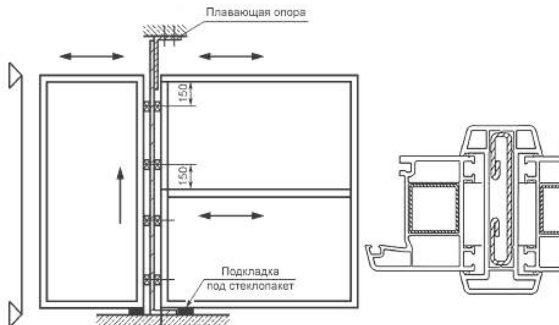
Рисунок Г.11 — Деформационный температурный шов
