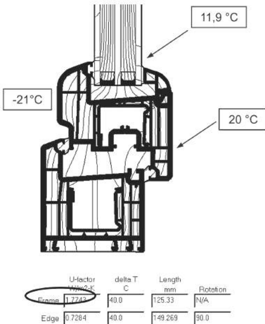
Рисунок Д.2 — Пример теплотехнической оценки узла сопряжения ПВХ профиля со стеклопакетом 4-10Kr-4И-10Kr-4И и теплой дистанционной рамкой
