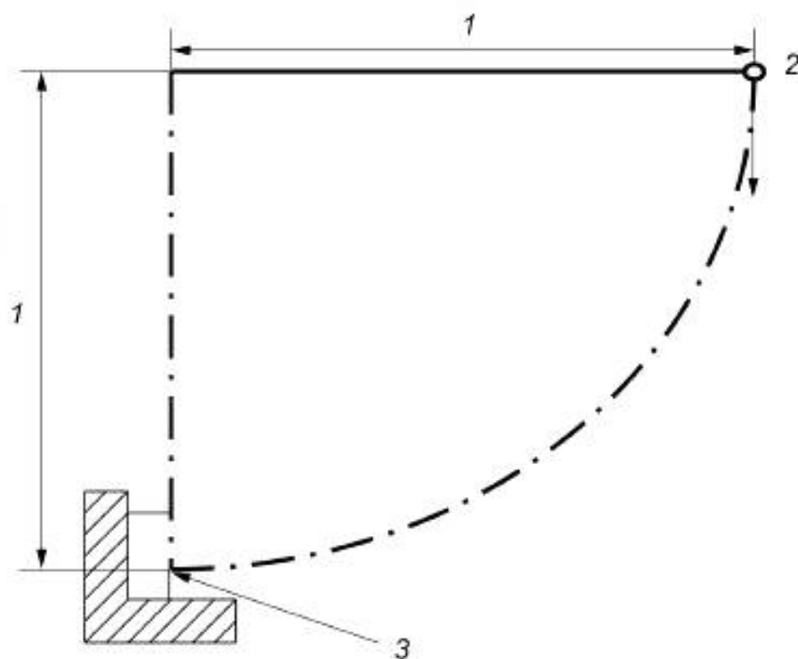
Схема движения маятника
