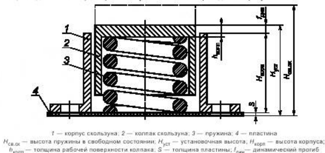
Рисунок А.1 — Схема и основные размеры скользуна типа ПКСПП
