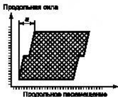
Рисунок 1 — Пример зависимости продольной силы от продольного перемещения
