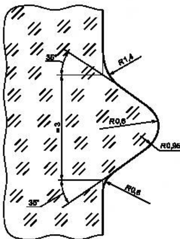
Рисунок 1 — Фрагмент профиля резьбы
