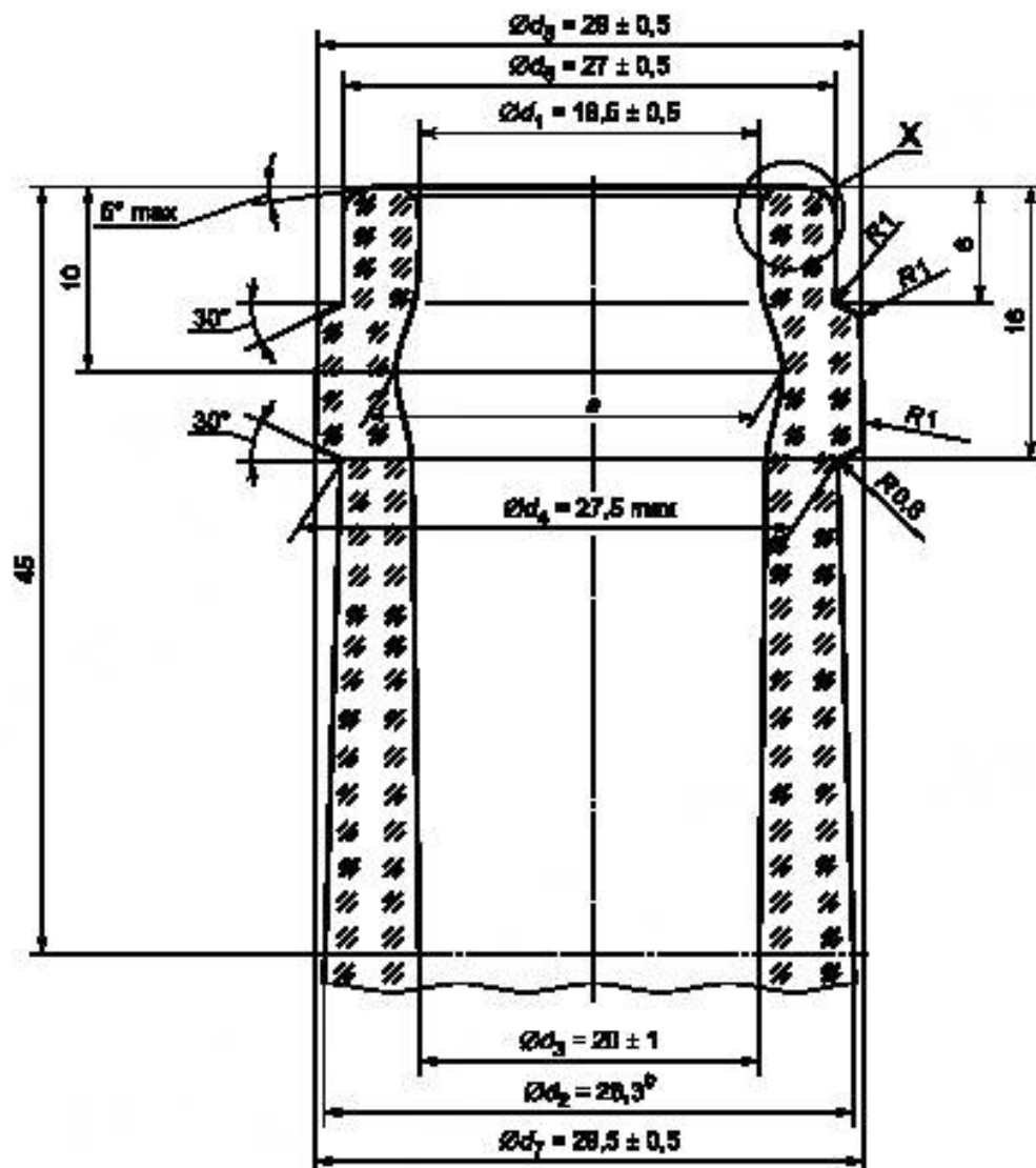
Рисунок 1 — Венчик горловины под корковую пробку с выходным диаметром 18,5 мм
