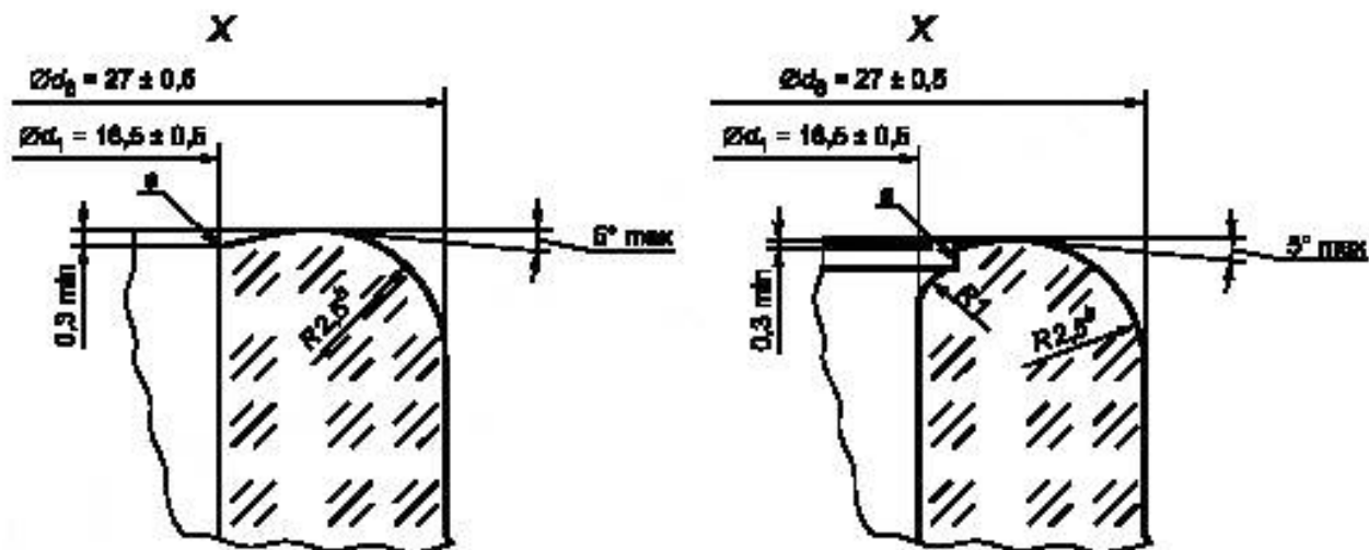
Рисунок 2 — Деталь горловины X
