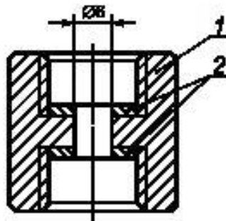
1 — переходник; 2 — прокладка
