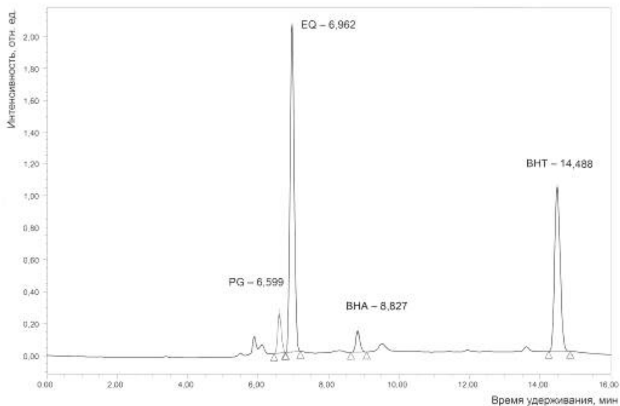
Рисунок А.3 — Хроматограмма экстракта кормовой добавки, полученная на колонке 1 (см. А.1)
