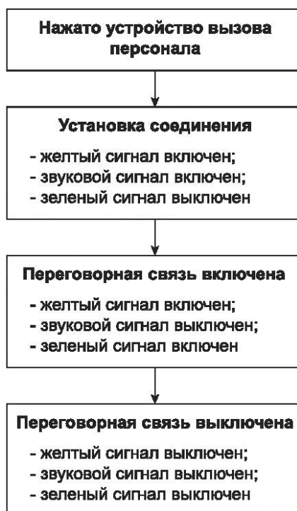
Рисунок 1 — Алгоритм формирования визуальных и звуковых сигналов
