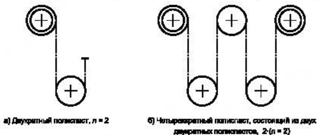
Рисунок С.3 — Полиспасты
