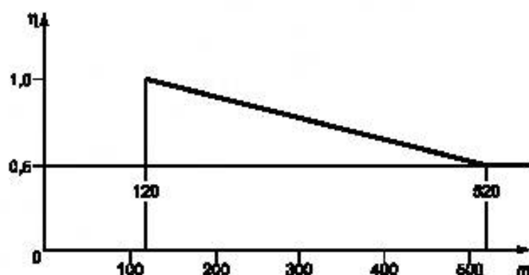
Рисунок 3 — Спектральный коэффициент нагрузки
