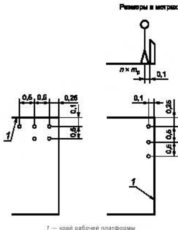
Рисунок 1 — Номинальная нагрузка (масса человека)
