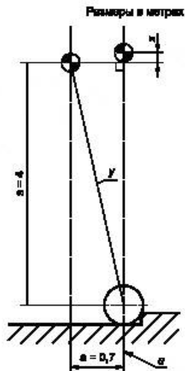
Рисунок Е.3 — Потенциальная энергия
