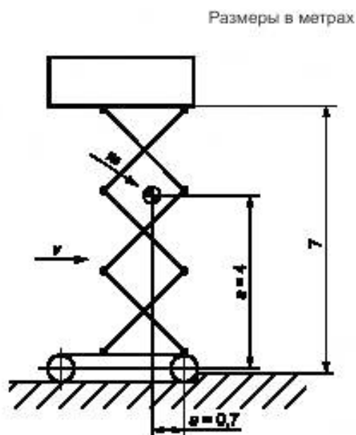
Рисунок Е.1 — МПРП перед препятствием
