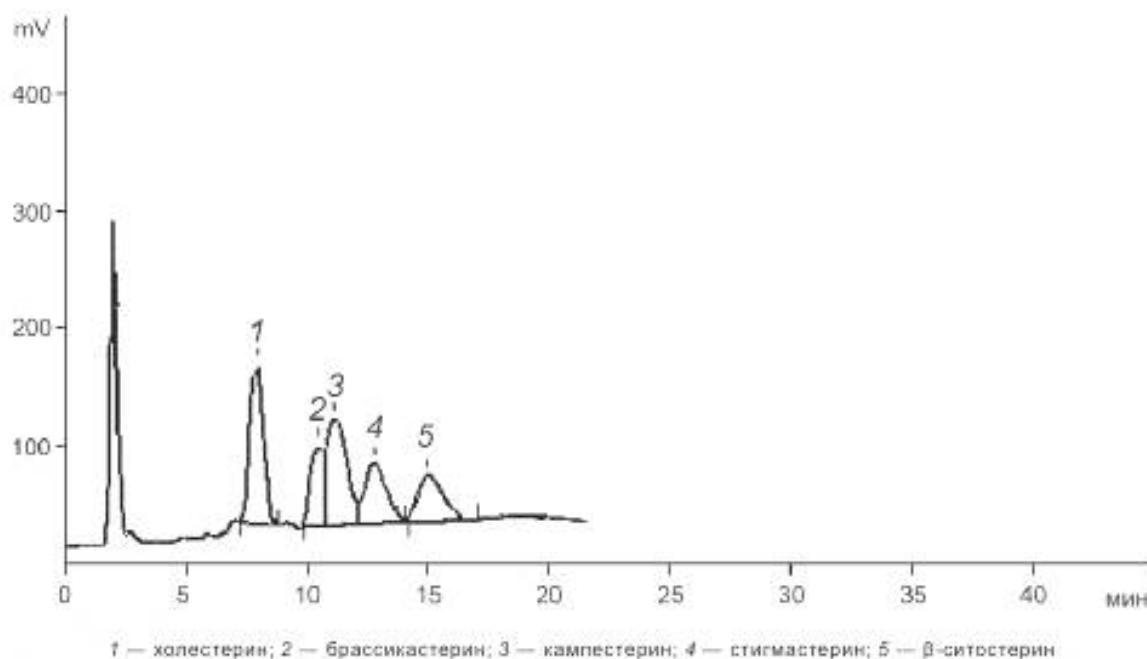
Рисунок 1 — Хроматограмма смеси стандартов стерина
