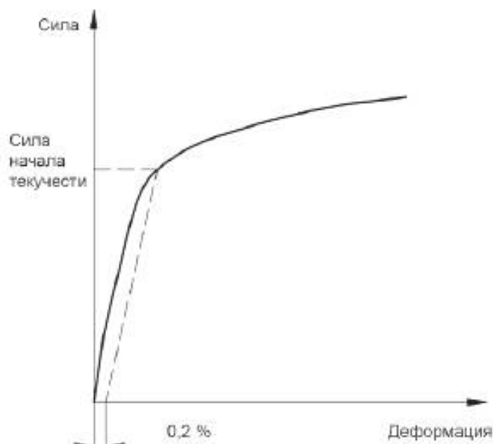
Рисунок 2 — Определение силы начала текучести
