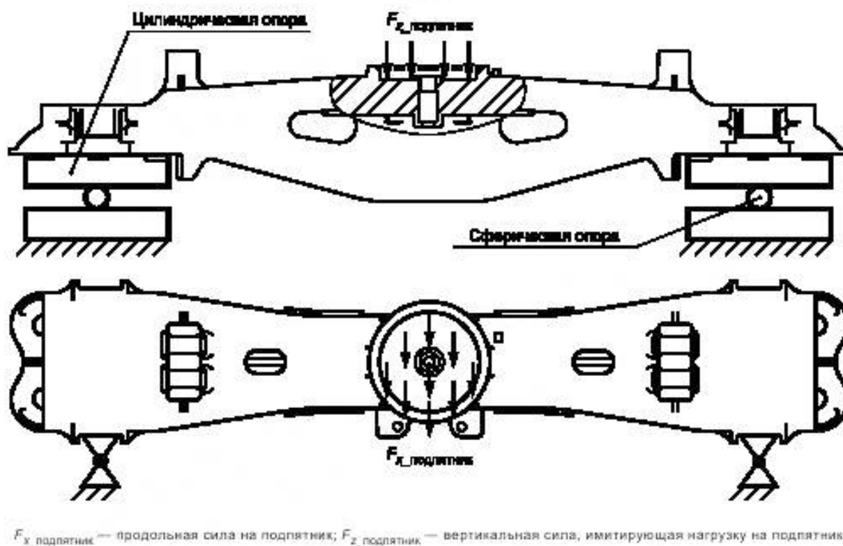
Рисунок 3 — Схема приложения сил к надрессорной балке
