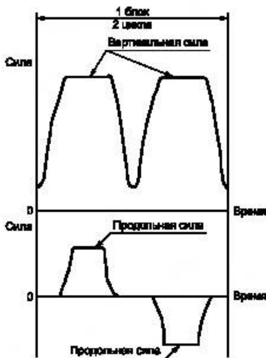
Рисунок 4 — Один блок приложения сил к надрессорной балке
