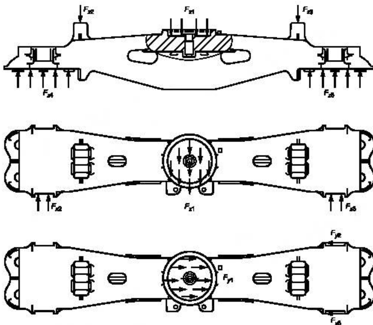
Рисунок 1 — Схема сил, действующих на надрессорную балку
