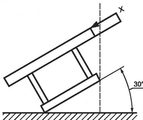
X — наиболее удаленный край верхней части сиденья-колыбель
