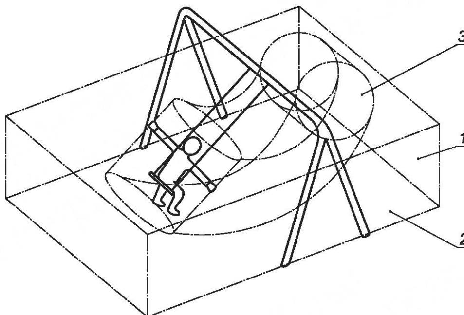
Рисунок 12 — Свободное пространство, пространство падения и зона приземления качелей
