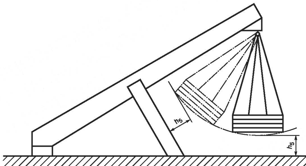
Рисунок 6 — Пример свободного пространства под сиденьем для качелей типа 3
