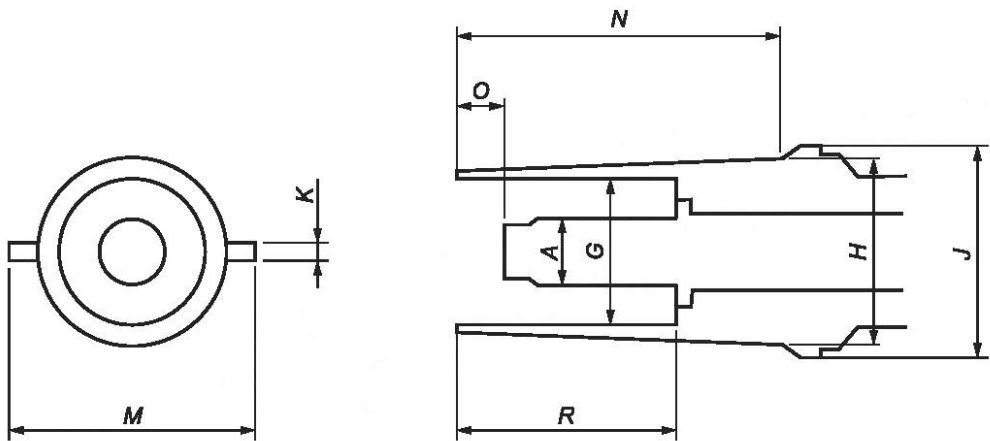
Размеры в миллиметрах
