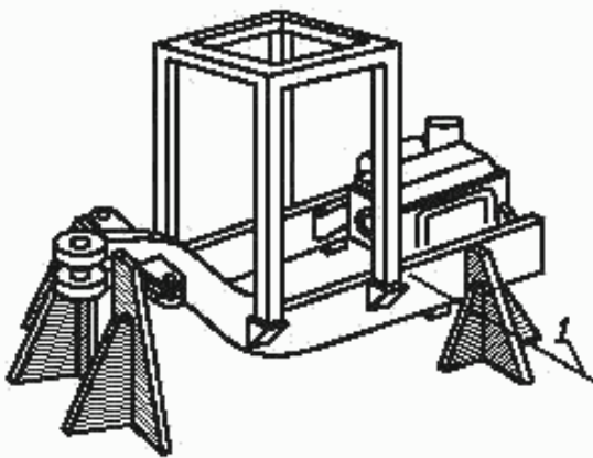
Рисунок 9 — Закрепление полурамы шарнирно-сочлененной машины
