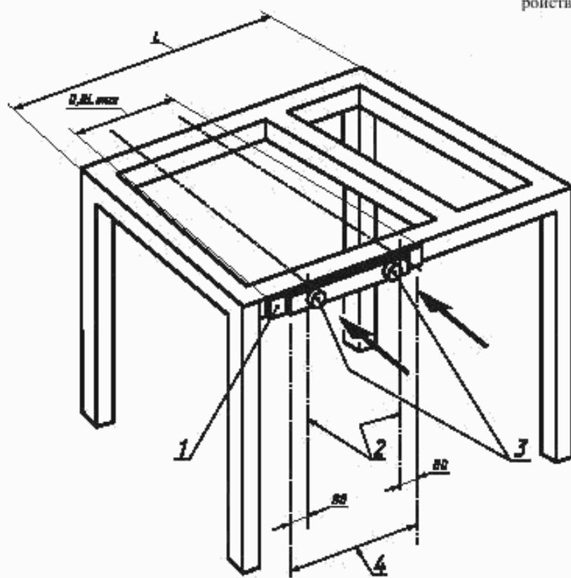
Рисунок 4 — Точка приложения боковой нагрузки к четырехстоечному ROPS
