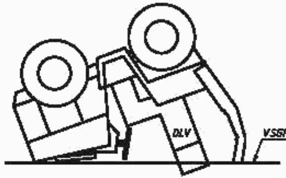
Рисунок 2 — Проникновение вертикальной имитируемой плоскости грунта VSGP в DLV
