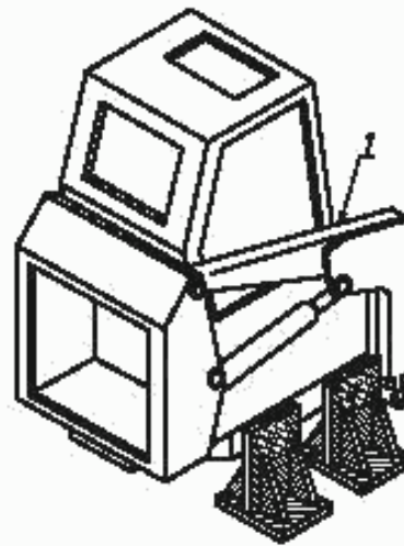
Рисунок 10 — Закрепление погрузчика с бортовым поворотом
