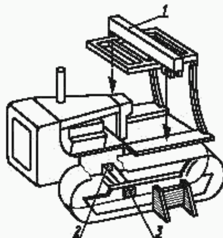
1 — балка для вертикального нагружения; 2 — заблокировано для предотвращения перемещения; 3 — блокировка противоблажающих трактов гусениц
