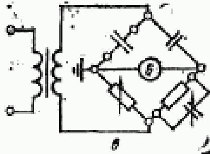
Схема с заземленной диагональю
