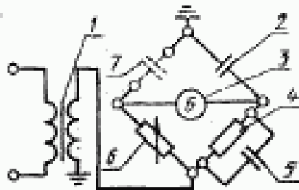
Перевернутая схема
