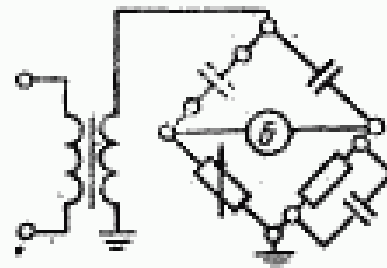
Нормальная схема
