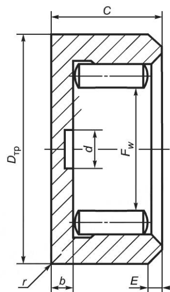
Рисунок 2 — Роликовый игольчатый карданный подшипник с фаской на наружном диаметре без галтели на доннышке
