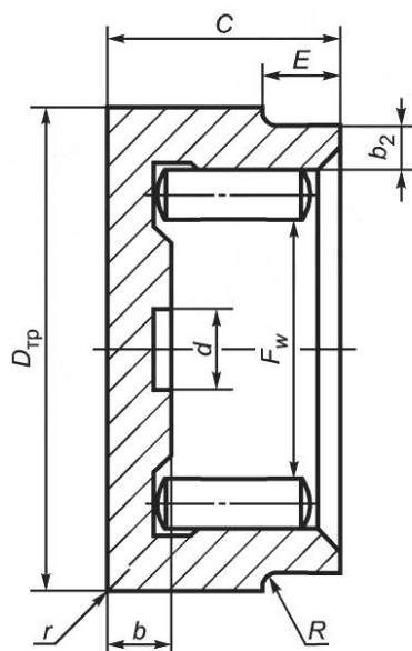
Рисунок 1 — Роликовый игольчатый карданный подшипник с радиусом на наружном диаметре и галтелью на доннышке
