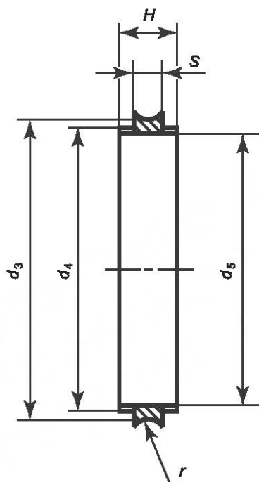
Рисунок 5 — Центрирующее кольцо
