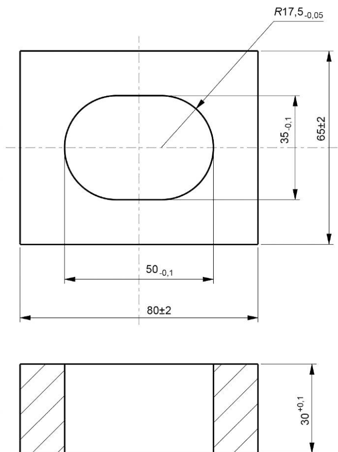
Рисунок 6 — Испытательный шаблон 1
