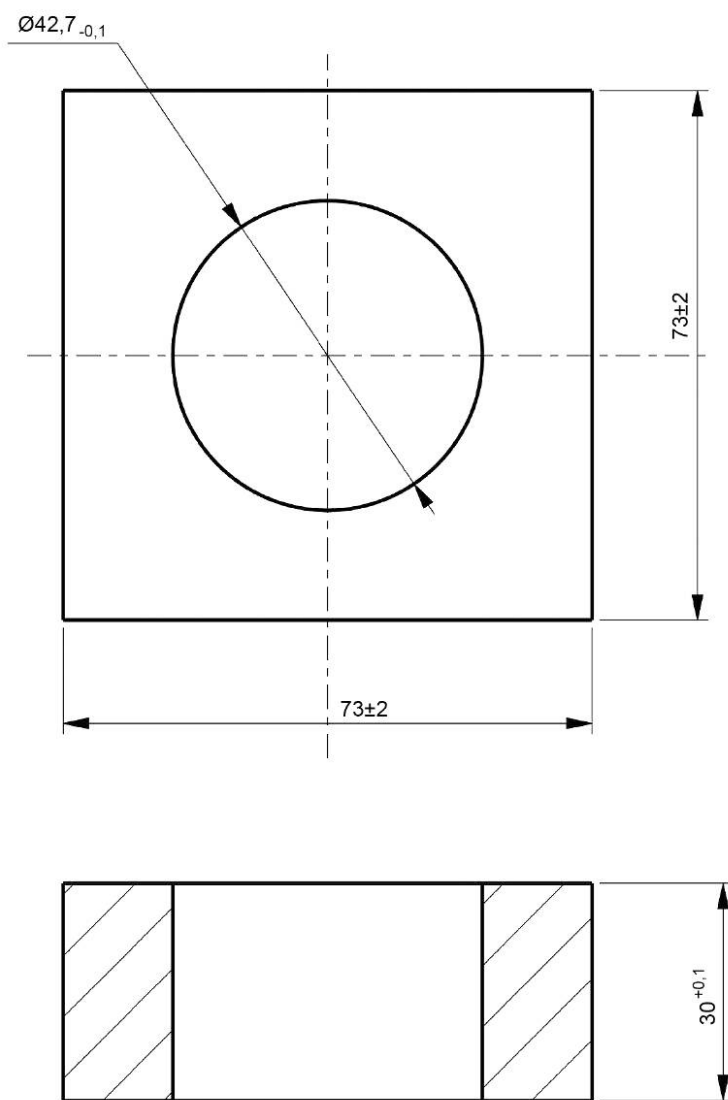
Рисунок 7 — Испытательный шаблон 2
