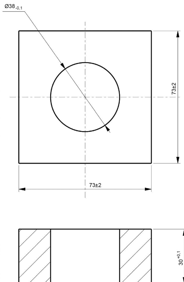
Рисунок 8 — Испытательный шаблон 3
