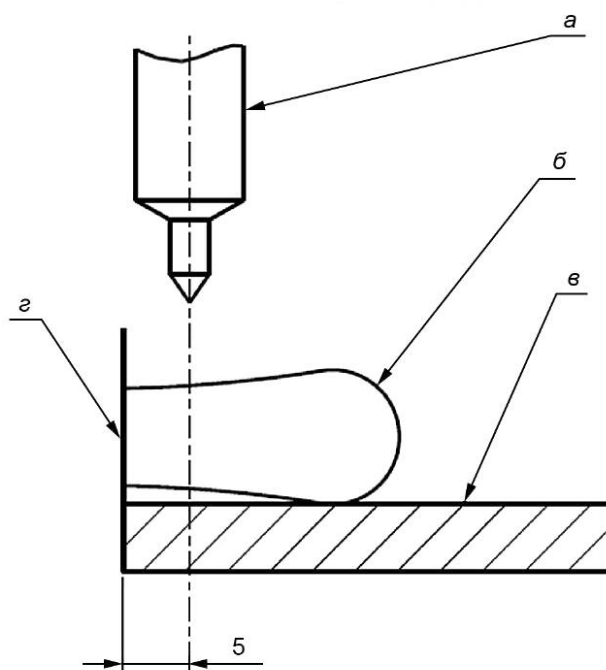
а — инструмент для прокола (см. 5.4); б — баллончик; в — упорная доска (см. 5.5); г — упор для режущей кромки баллончика
