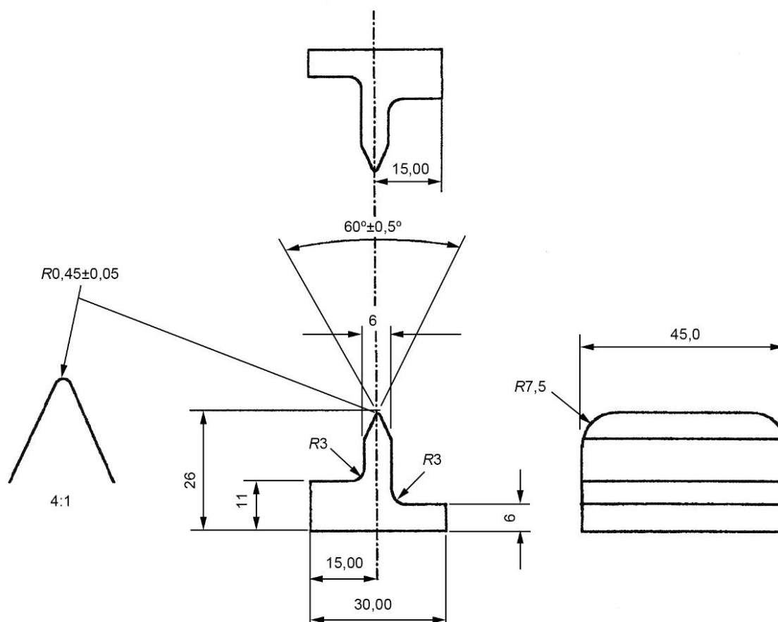
Рисунок 4 — Верхний и нижний зажимы определения прочности
