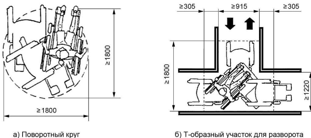
Рисунок 1 — Устройство поворотного круга и Т-образного участка
