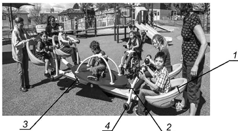
1 — сиденье; 2 — поручень; 3 — балансир; 4 — опора с демпфером
