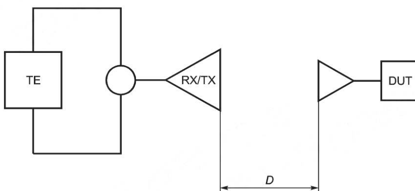
Рисунок 1 — Испытательный стенд с двумя антеннами
