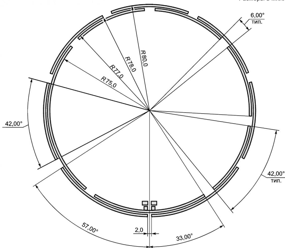
Рисунок С.1 — Конструкция антенны, которая будет использоваться для измерений индуктивных радиочастотных меток УВЧ
