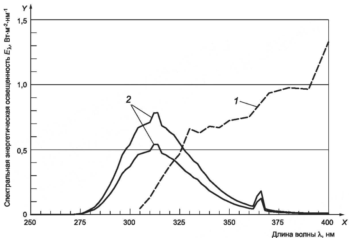
Рисунок А.3 — Спектральная энергетическая освещенность для типовых ламп типа 2 (UVB-313) в сравнении с дневным светом по таблице 4 документа [2]
