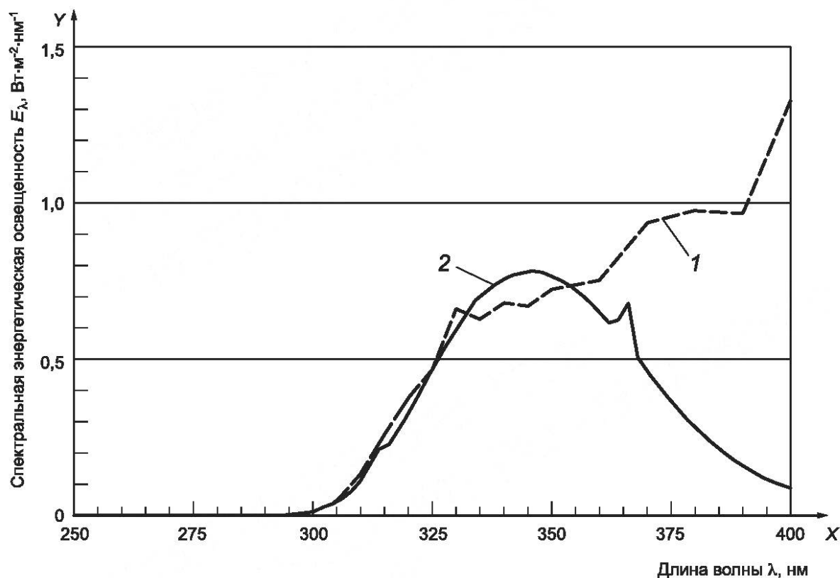
Рисунок А.1 — Спектральная энергетическая освещенность для типовых ламп типа 1А (UVA-340) в сравнении с дневным светом по таблице 4 документа [2]
