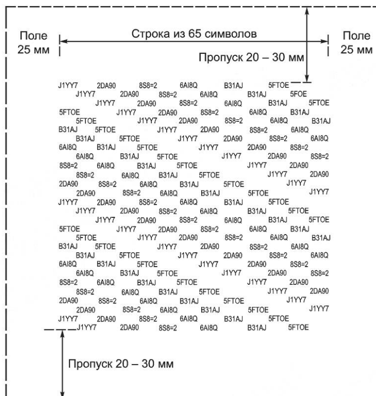
Рисунок DA.2 — Пример испытательного шаблона при длине строки 65 символов
