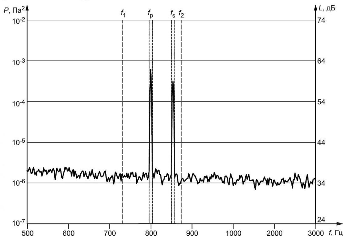
Рисунок D.3 — Применение метода тон/шум к нескольким тонам в критической полосе
