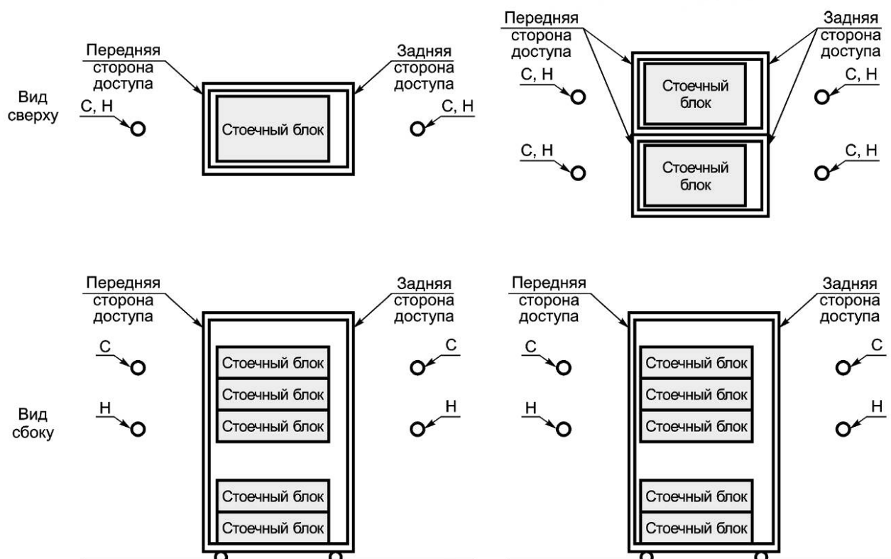
Рисунок ДА.7 — Пример расположения оператора в положениях «стоя» (С) и «нагнувшись» (Н) для стоечных систем, содержащих стойечные блоки
