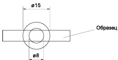
Рисунок 20 — Определение частей изоляционного материала, подлежащих испытанию, — схематическое изображение (см. 24.1)
