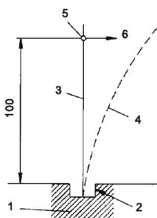
Рисунок 10а — Принцип действия испытательной установки для испытания на отклонение безвинтовых зажимов
