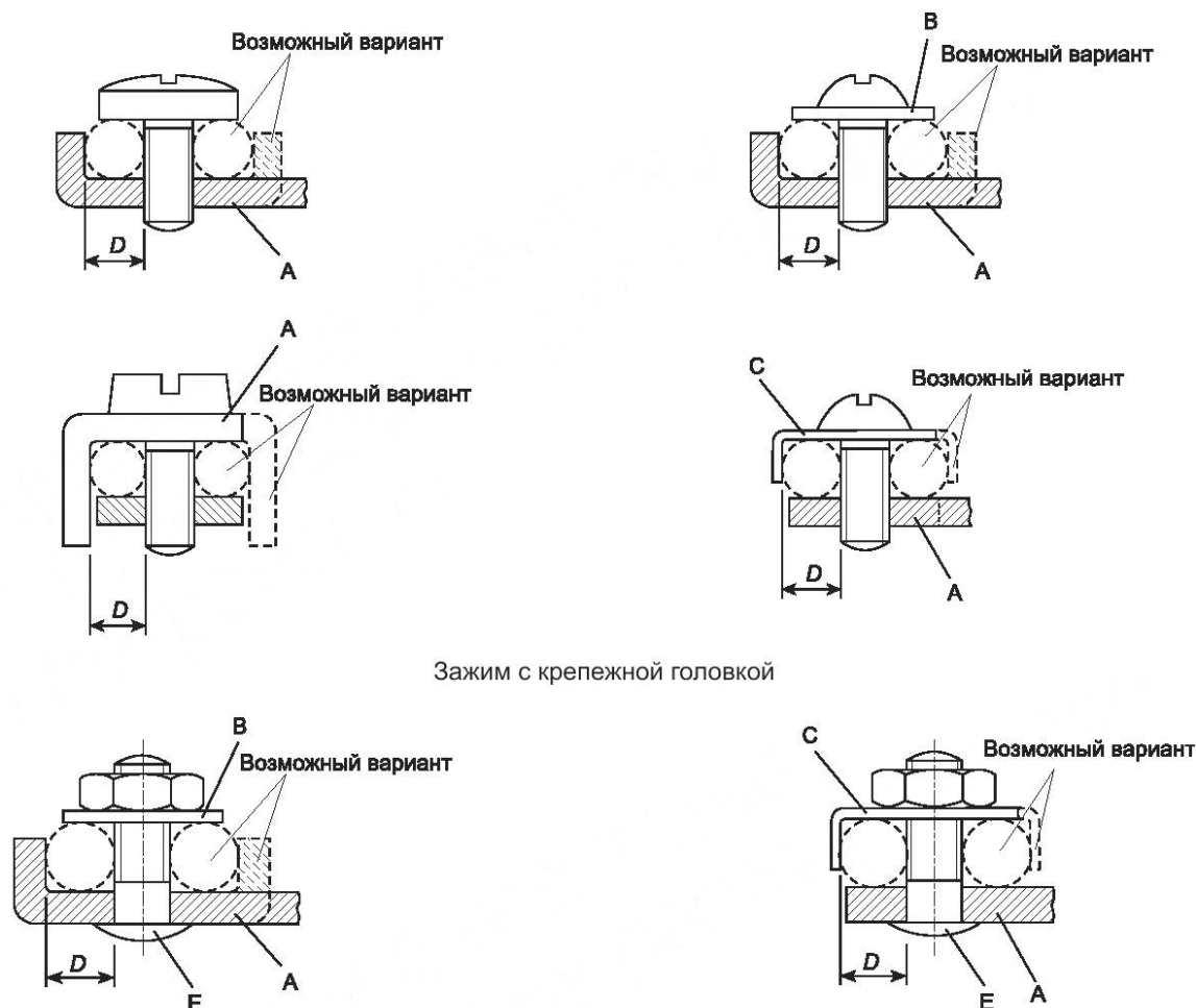
Зажим с крепежной гайкой
