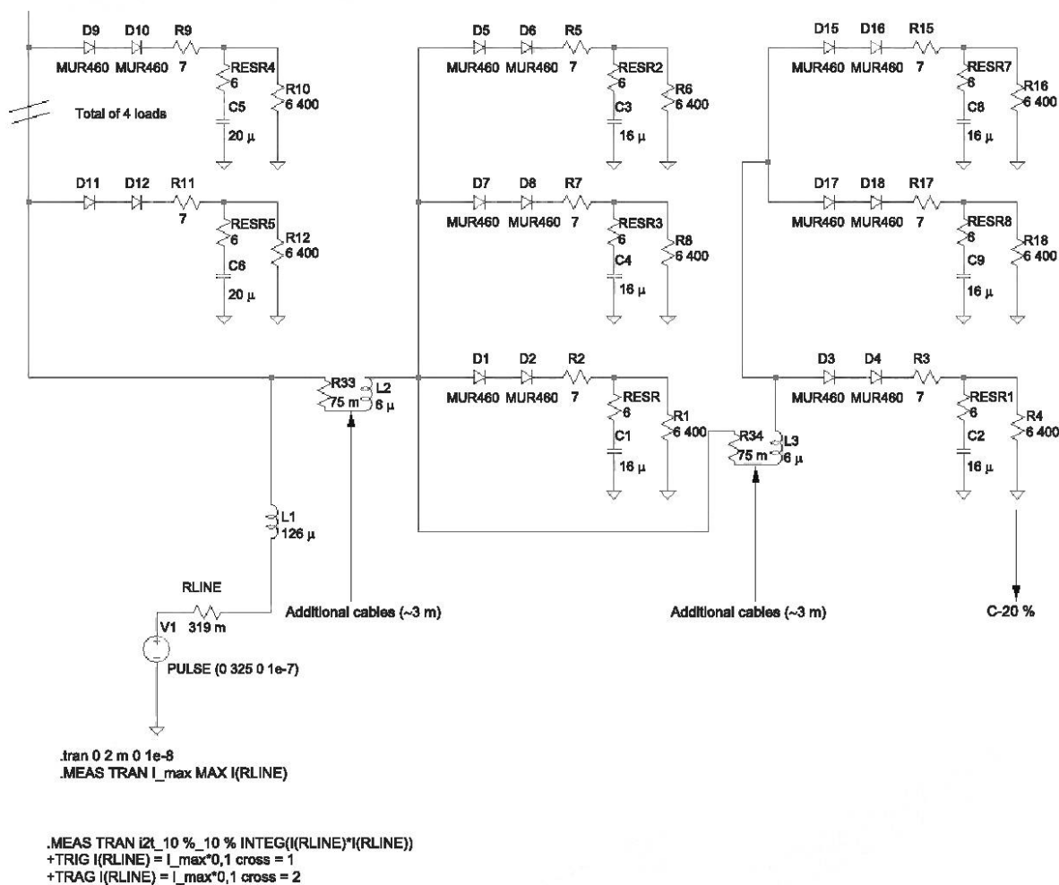
Рисунок С.3 — Модель для включения нескольких ламп
