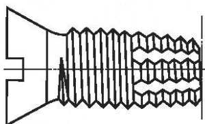
Рисунок 7 — Самонарезающий режущий винт
