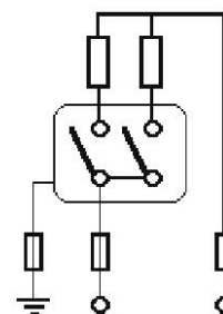
Выключатель по схеме 5
