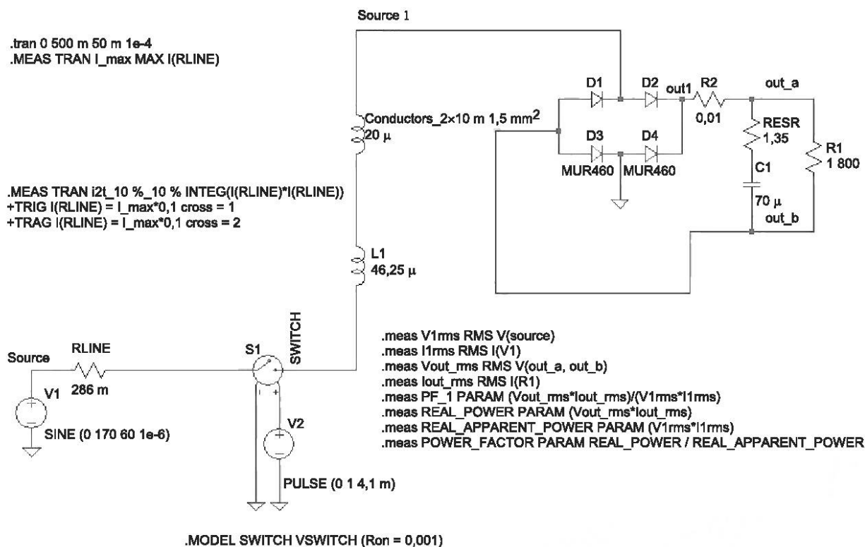
Рисунок С.1 — 120 В 15 Вт (модель LT spice)
