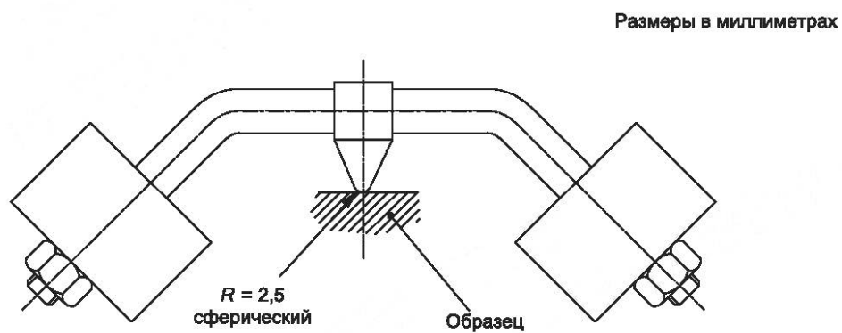
Рисунок 19 — Аппарат шарико-прижимной
