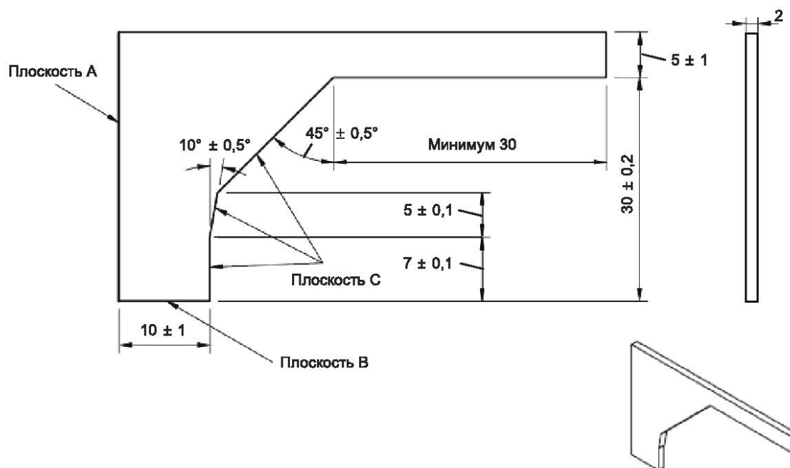
Рисунок 14 — Калибр (толщина около 2 мм) для проверки контуров крышек, накладок или исполнительных элементов
