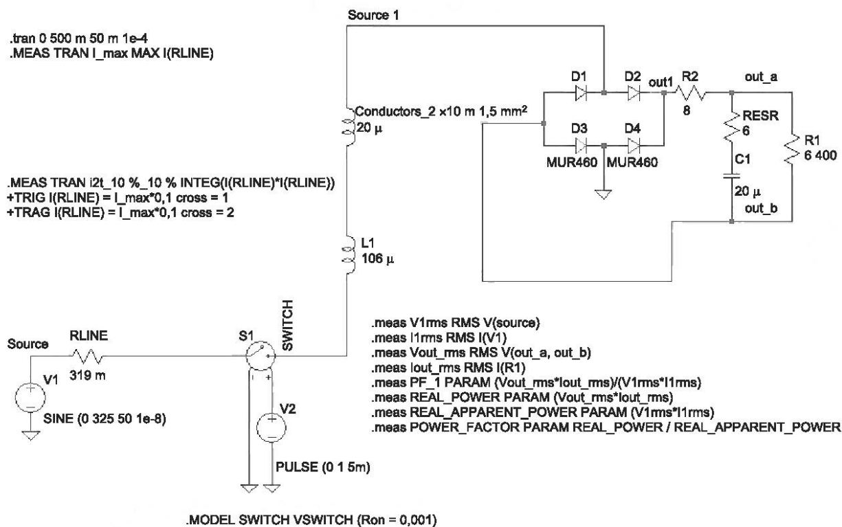
Рисунок С.2 — 230 В 15 Вт (модель LT spice)
