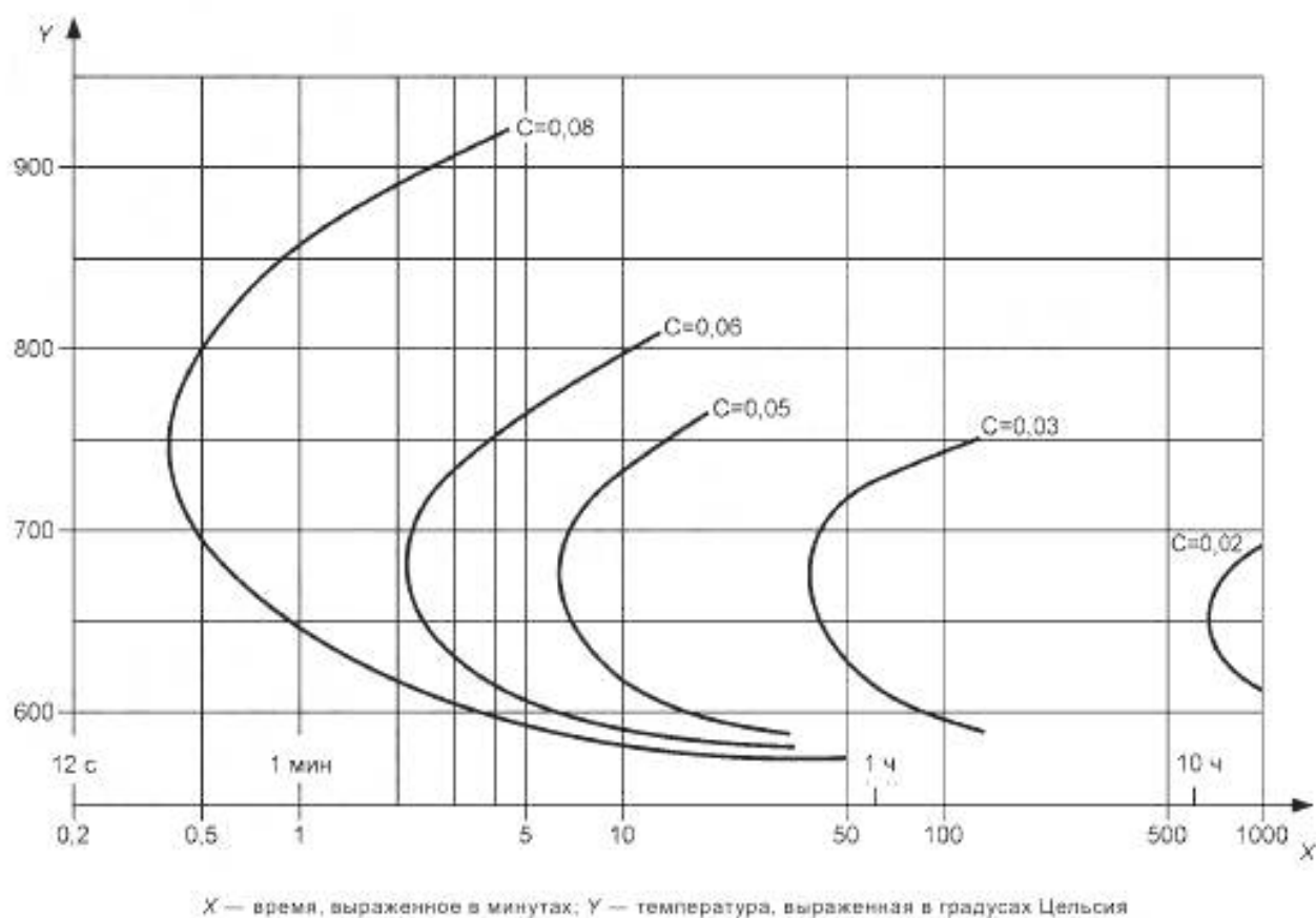
Рисунок F.1 — Температурно-временная диаграмма межкристаллитной коррозии в аустенитной нержавеющей стали марки А2
