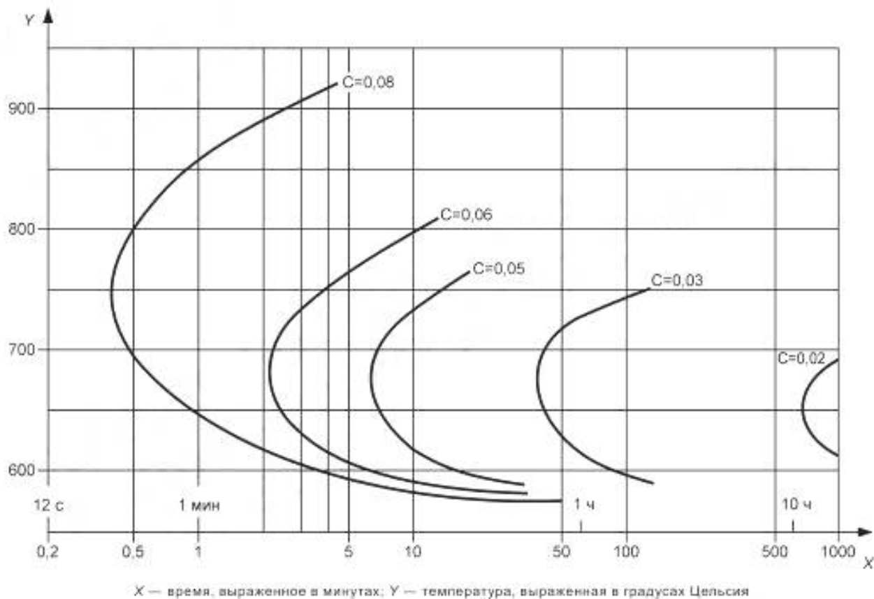
Рисунок D.1 — Температурно-временная диаграмма межкристаллитной коррозии в аустенитной нержавеющей стали марки А2
