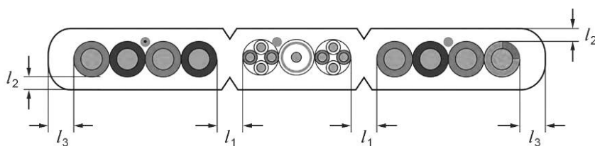
Рисунок 4 — Поперечное сечение кабеля с обозначением толщин оболочки и перемычек между группами жил
