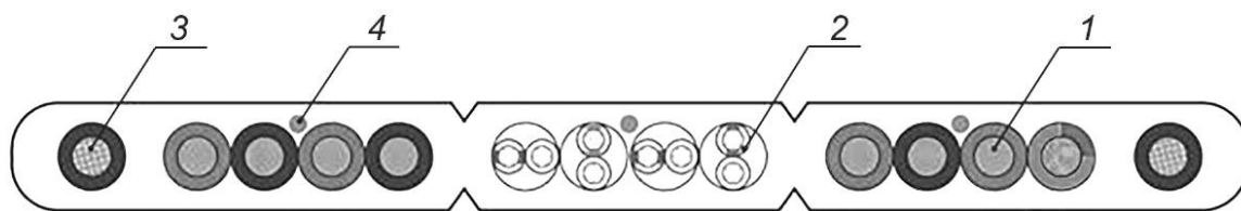
1 — основные изолированные жилы; 2 — элементы передачи сигналов (скрученные пары); 3 — усиливающие элементы; 4 — вспарывающая нить
