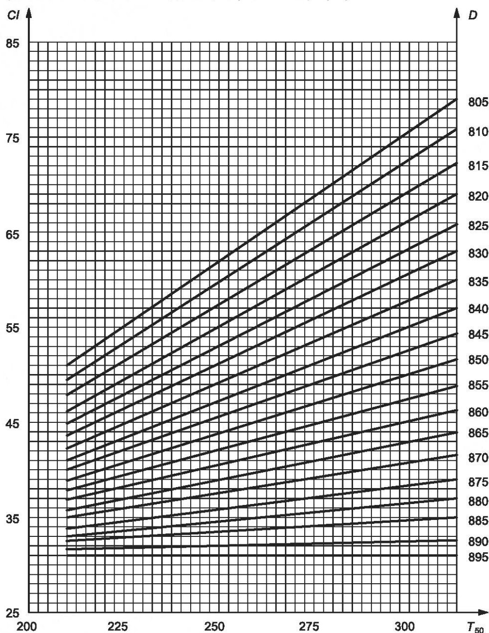
Рисунок А.1 — Номограмма предварительной оценки цетанового индекса на основе значений плотности при температуре 15 °С и температуры, при которой перегоняется 50 % об.
