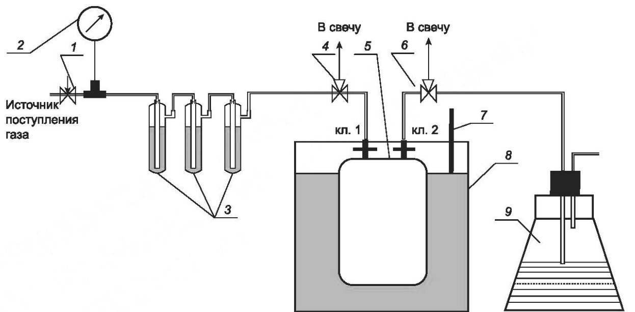
1 — газовый редуктор/выход газопровода; 2 — манометр газового редуктора; 3 — увлажнитель газа; 4, 6 — краны соединительные трехходовые; 5 — калориметрическая бомба; 7 — средство измерения температуры; 8 — термостат; 9 — склянка (счетчик пузырьков)
