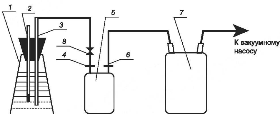
1 — коническая колба; 2 — средство измерения температуры; 3 — трубка; 4 и 6 — заправочные клапаны; 5 — калориметрическая бомба; 7 — склянка Вульфа; 8 — закрывающий кран
