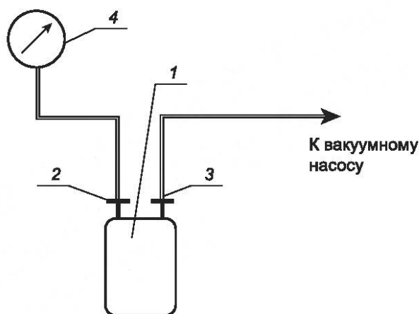
1 — калориметрическая бомба; 2 и 3 — заправочные клапаны; 4 — вакуумметр
