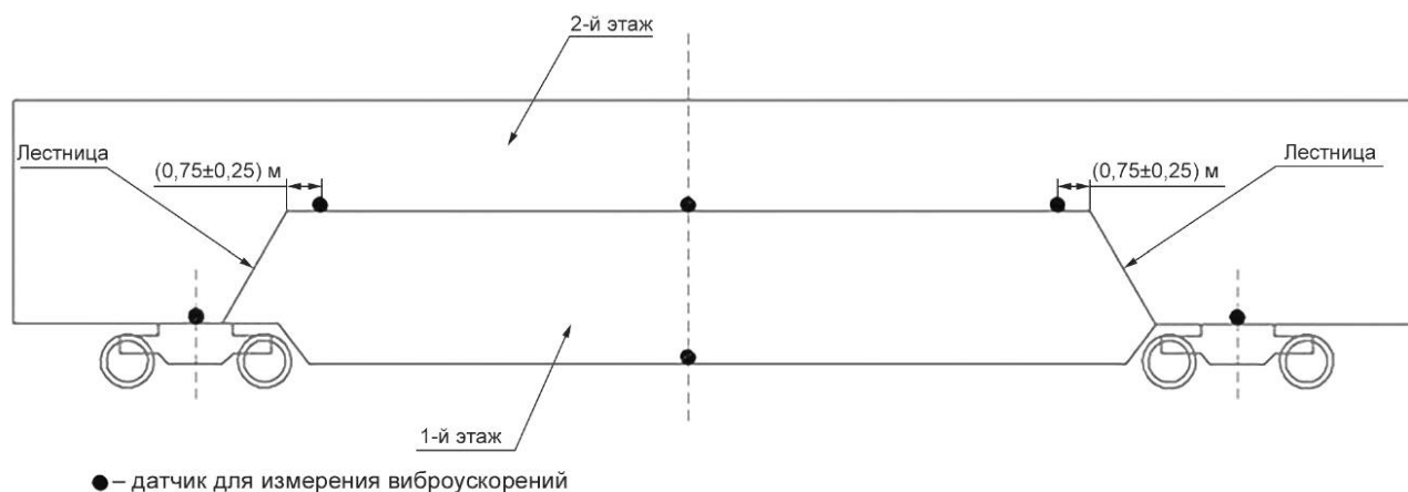
Рисунок 1 — Схема расположения датчиков для определения виброускорений на двухэтажном вагоне
