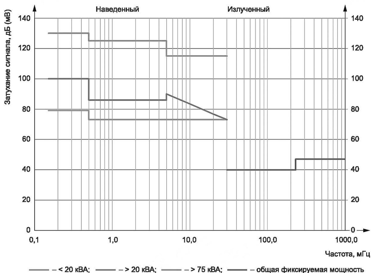
Рисунок 4 — Пределы класса А (квазипиковые) для проводимого и электромагнитного излучения на расстоянии 10 м по ГОСТ CISPR 11
