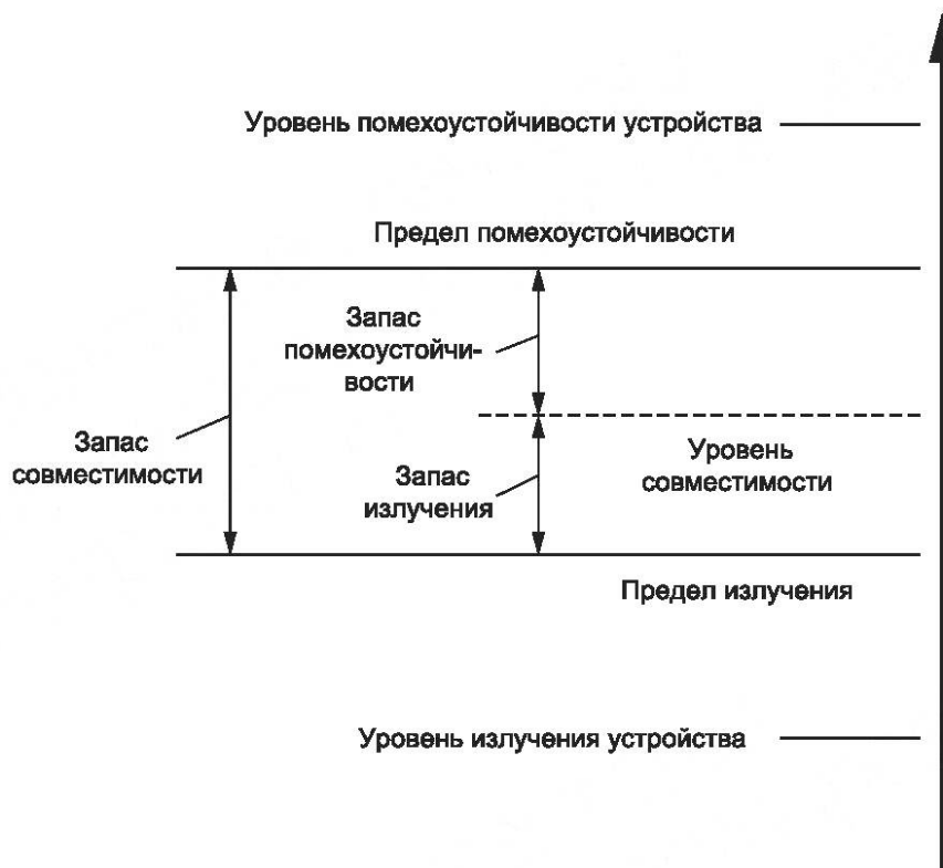
Рисунок 3 — Принцип ЭМС
