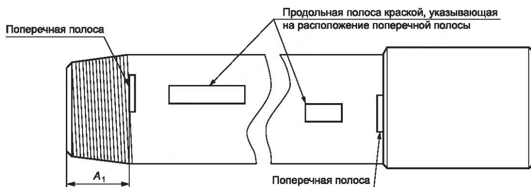
д) Знак свинчивания в виде поперечной полосы на трубах с резьбовым соединением BC
