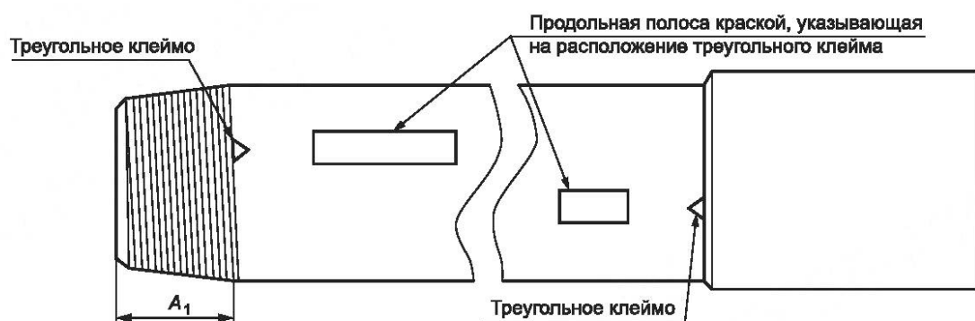
б) Знак свинчивания в виде треугольного клейма на трубах с резьбовым соединением BC
