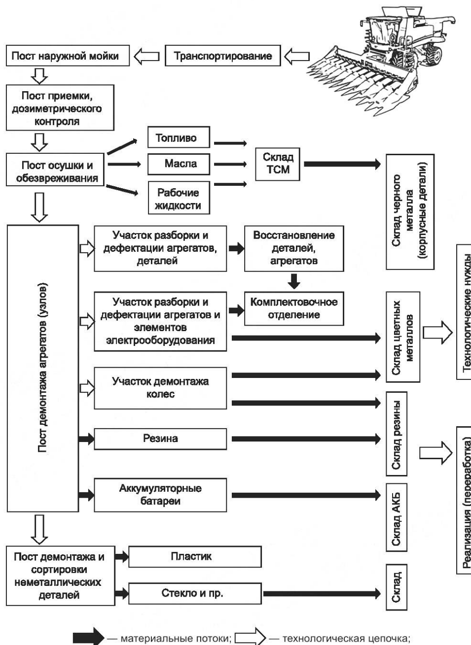
Рисунок Д.1 — Вариант технологической структуры предприятия по утилизации комбайнов
