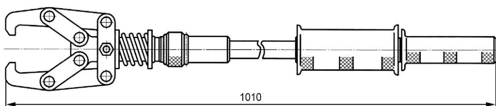
Рисунок Д.6 — Инерционный съемник (СКНТЦ ГОСНИТИ 000000. 003)
