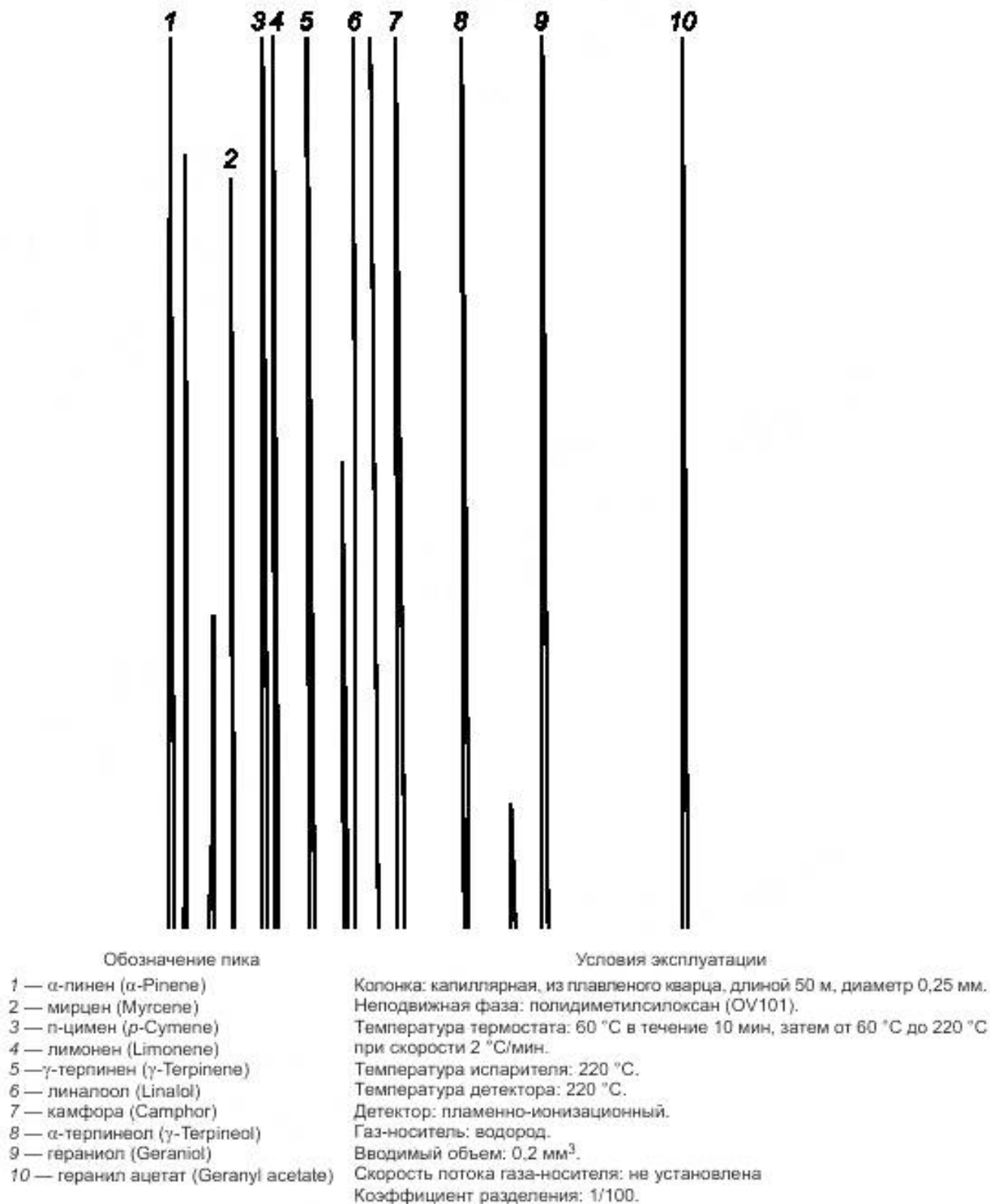
Рисунок А.1 — Типичная хроматограмма, полученная на неполярной колонке
