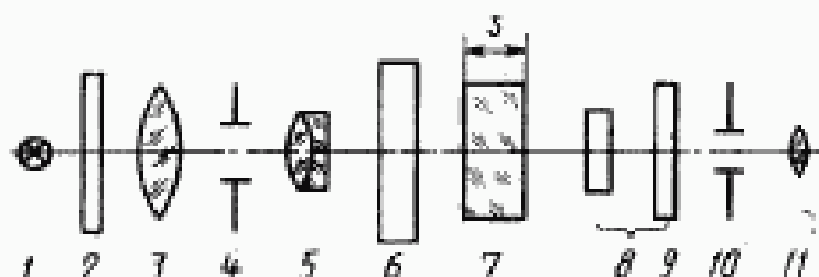
1 — источник излучения; 2 — светофильтр; 3 — конденсор; 4, 10 — диафрагмы; 5 — объектив коллиматора; 6 — волновод; 7 — измеримый образец оптического материала; 8 — компенсатор; 9 — анализатор; 11 — окуляр
