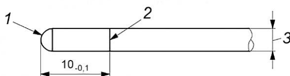
Рисунок 1 — Шаблон пальца с полусферическим торцом
