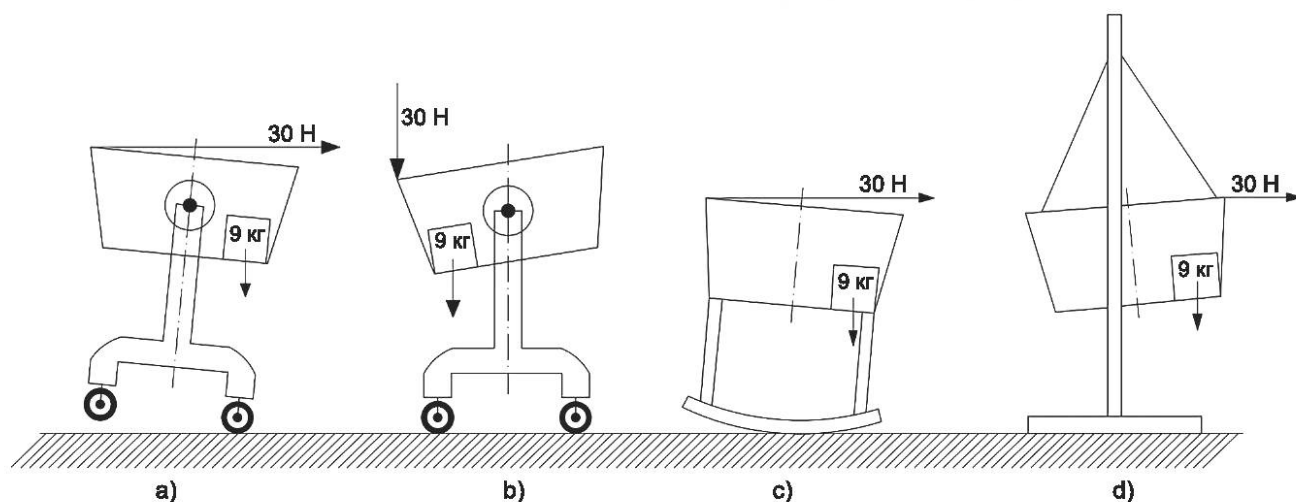
a), b) — колыбели на ножках, в т. ч. с колесами; c) — колыбель на изогнутых полозьях; d) — люлька
