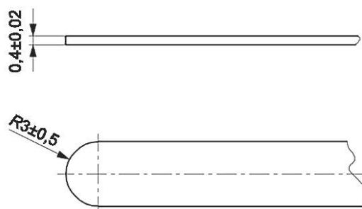
Рисунок 11 — Измерительный щуп
