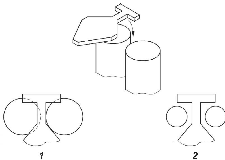
Рисунок 13 — Способы вставки части В шаблона
