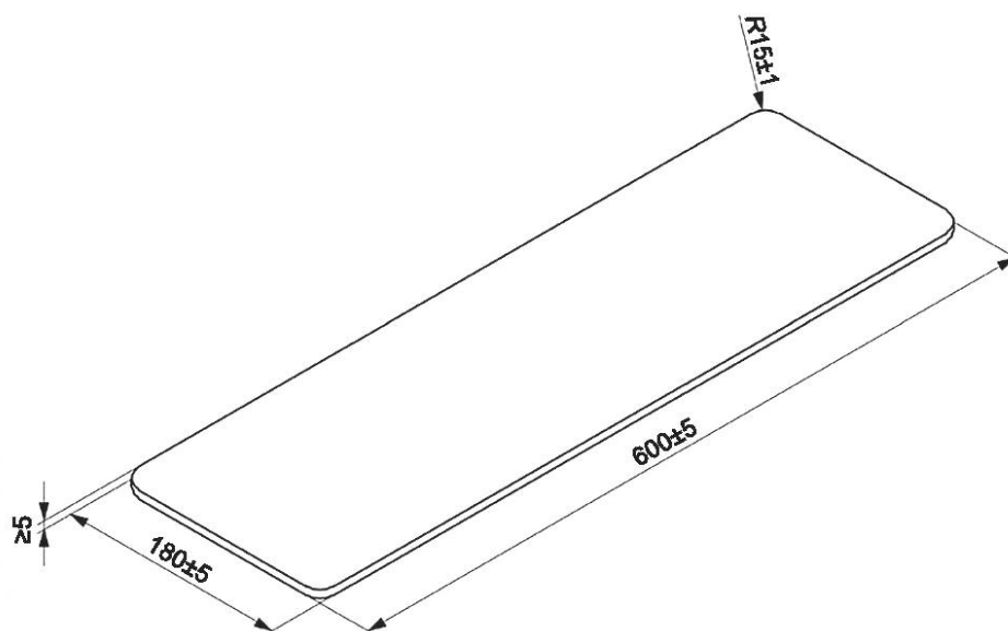
Рисунок 9 — Контрольная пластина
