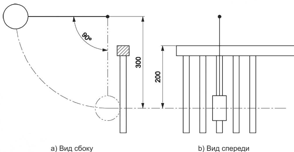
Рисунок 19 — Испытание боковых ограждений на удар
