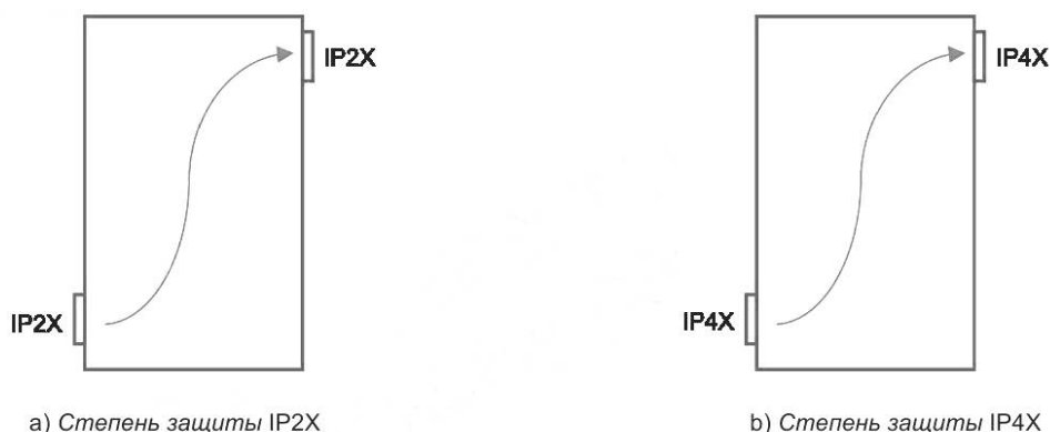
Рисунок В.1 — Примеры диагональной установки
