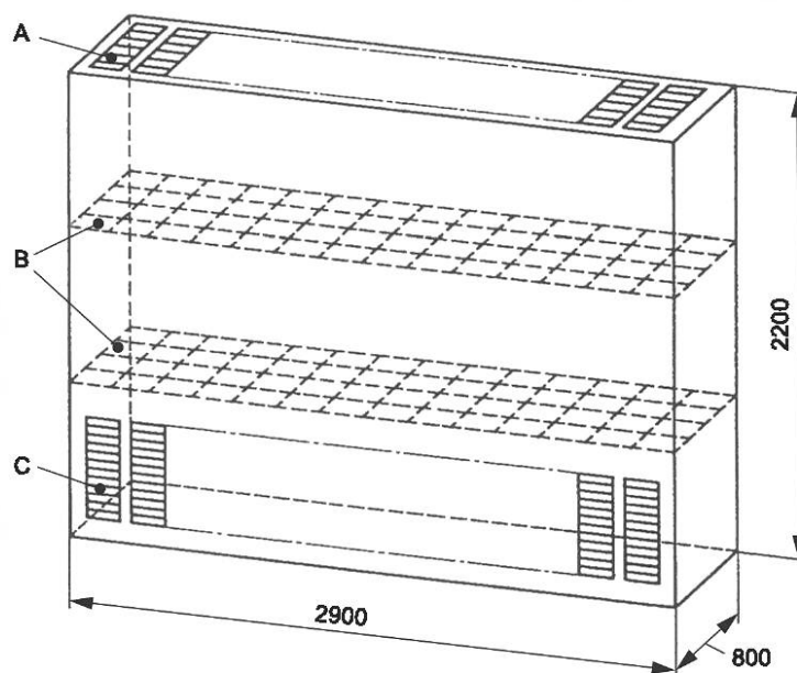
A — отверстия для отведения воздуха; B — горизонтальные перегородки с вентиляционными отверстиями, например, перфорированная пластина; C — отверстия для притока воздуха
