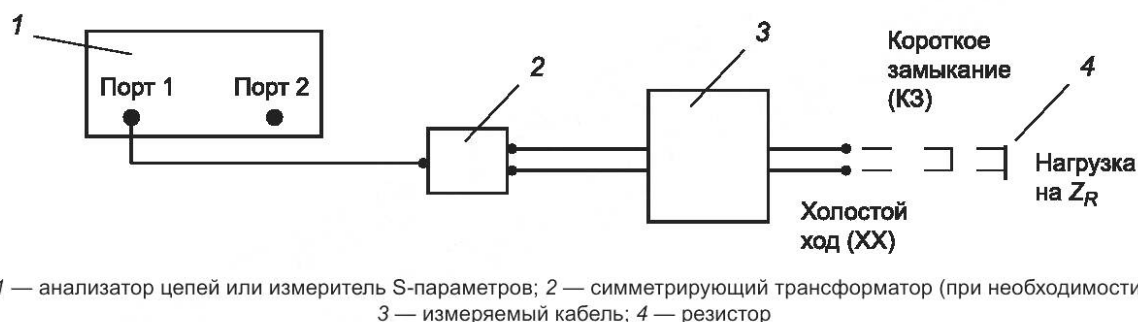
Рисунок 19 — Схема для измерения волнового и входного сопротивлений цепи кабеля и затухания отражения
