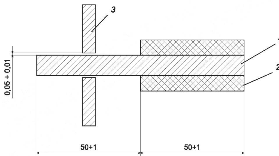
1 — токопроводящая жила; 2 — изоляция; 3 — металлическая пластина, жестко скрепленная с фиксированным (пассивным) зажимом разрывной машины
