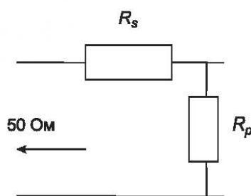
Рисунок 2 — Цепь согласования при Z_K менее 50 Ом
