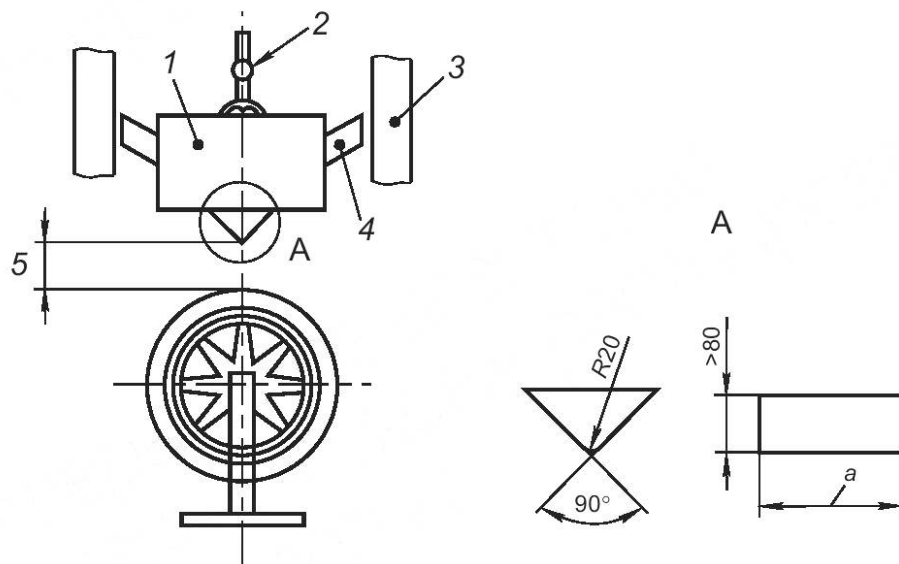
1 — груз; 2 — спусковой механизм; 3 — рама; 4 — направляющая; 5 — высота; удара; a = 1,5 \times ширина обода
