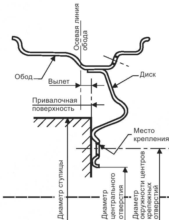
Рисунок 1 — Профиль колеса
