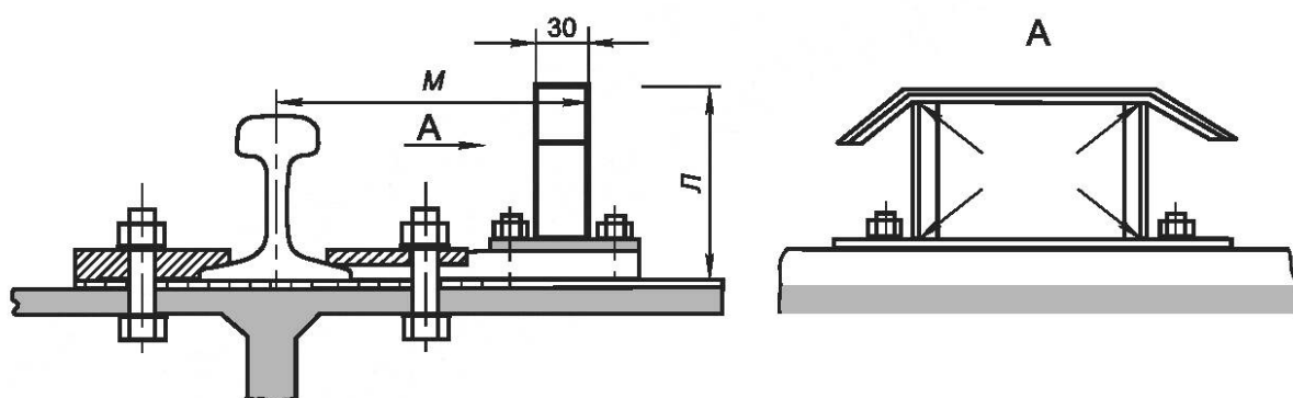
Рисунок В.3 — Типовая конструкция отключающей линейки
