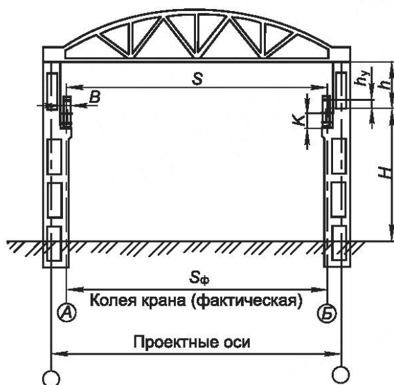
а) — пример для опорного крана
