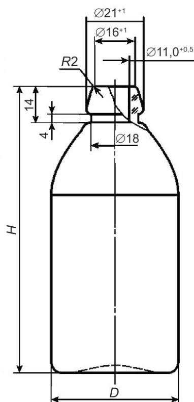
Рисунок 2 — Бутылка типа БТ-2
