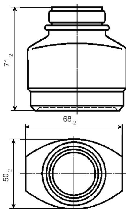
Рисунок 2 — Бутылка типа БТ-2
