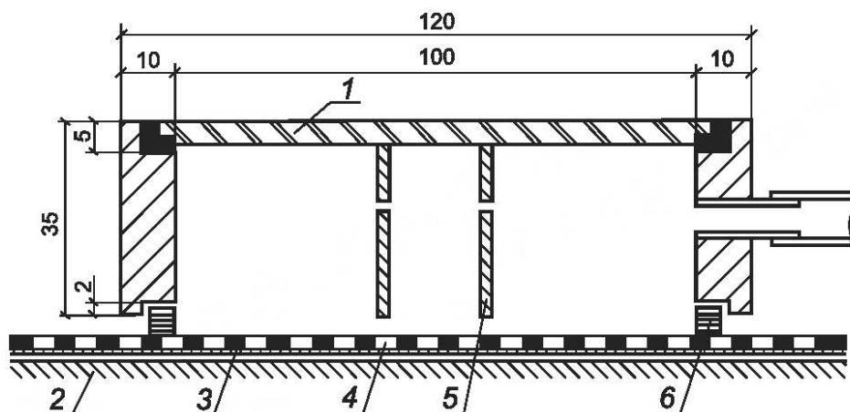
1 — стеклянная пластина; 2 — опорная стальная пластина; 3 — воздухопроницаемый слой; 4 — образец для испытаний; 5 — прозрачная пластиковая трубка; 6 — прокладка
