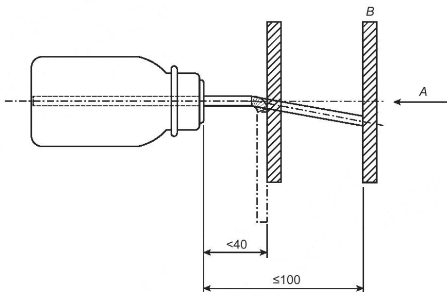
Рисунок 18 — Пример испытания на гибкость
