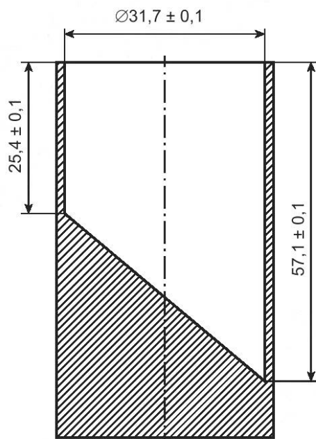
Рисунок 9 — Цилиндр для мелких деталей
