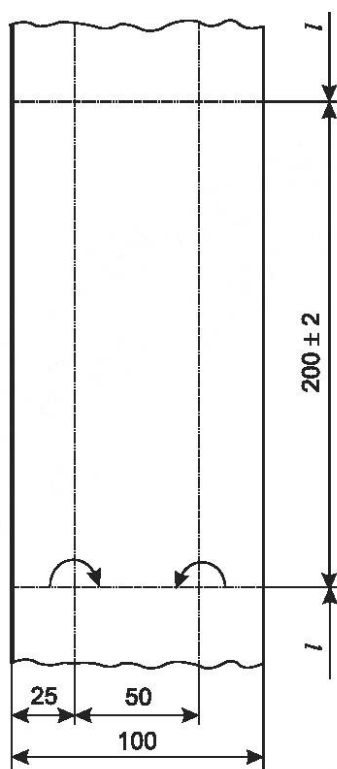
Рисунок Б.1 — Складывание образца для испытаний
