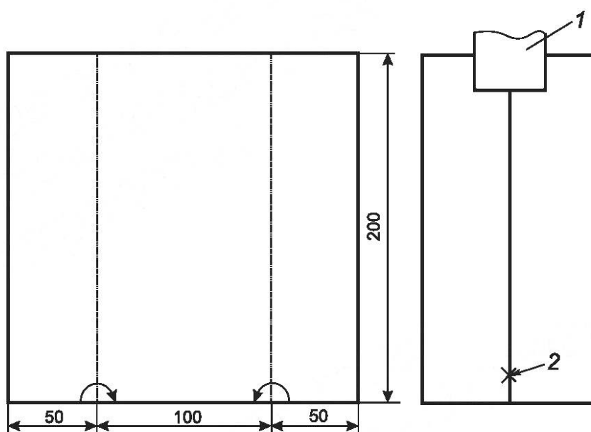
1 — верхний зажим; 2 — положение гвоздя
