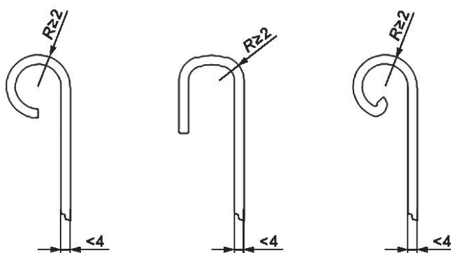
Рисунок В.2 — Примеры загнутых, скрученных и спиральных кромок
