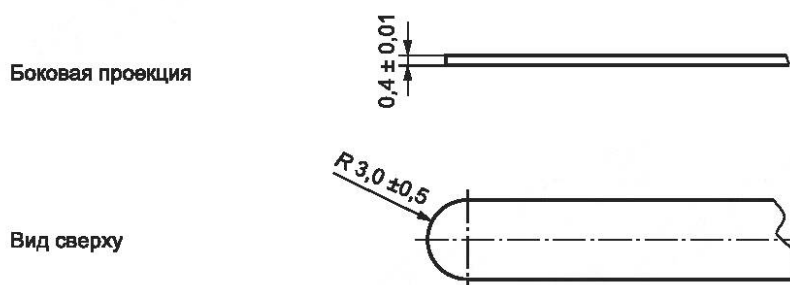
Рисунок 11 — Измерительный щуп
