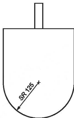
Рисунок 14 — Сбрасываемый ударник
