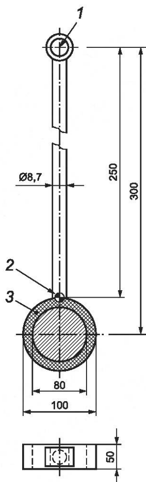
Рисунок 15 — Боковой ударник
