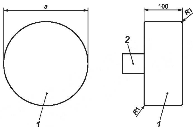
Рисунок 4 — Шаблон «большой головы» с держателем
