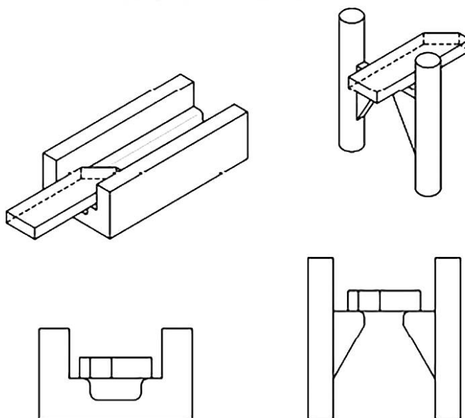
Рисунок 21 — Примеры опор на несплошном ограждении под углом менее 55^\circ
