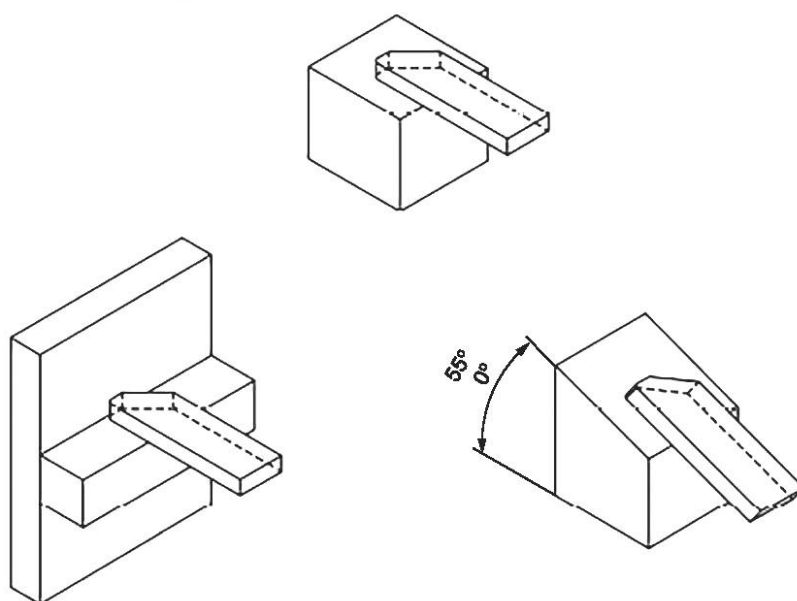
Рисунок 20 — Примеры опор на сплошном ограждении под углом менее 55°
