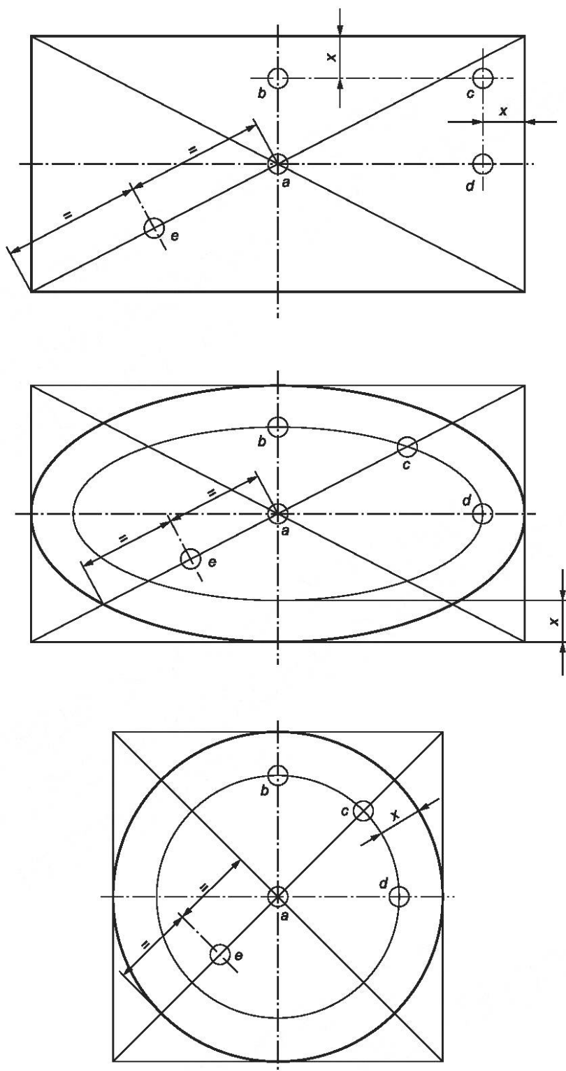
Рисунок 28 — Точки удара
