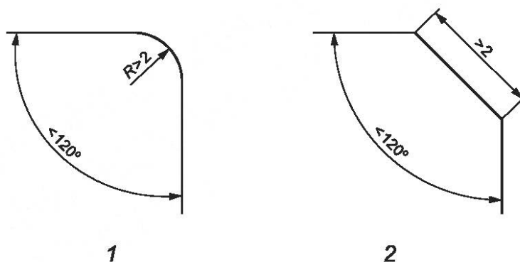
Рисунок В.1 — Примеры проектирования безопасных углов и кромок
